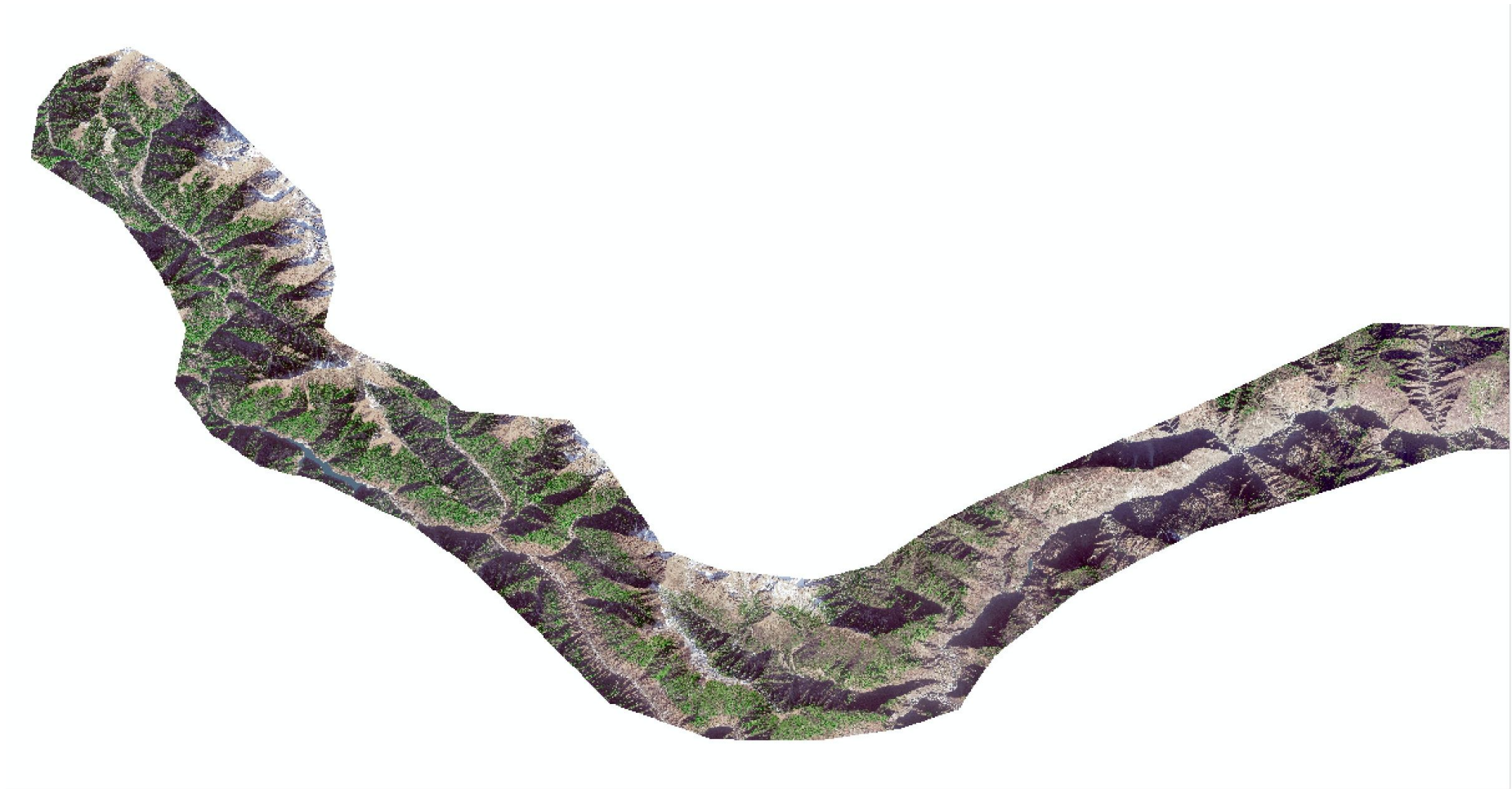
1-7 标遥感图像
