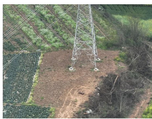
石门 N55 塔基施工场地平整
