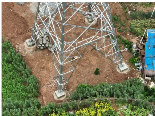
青龙坡 N40 塔基施工场地平整
