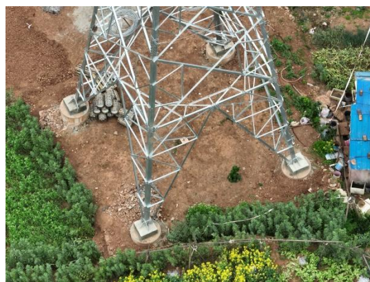
青龙坡 N40 塔基施工场地现状
