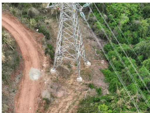
青龙坡 N12 塔基施工场地现状
