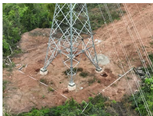
青龙坡 N5 塔基施工场地现状
