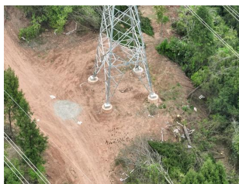
石门 N9 塔基施工场地现状
