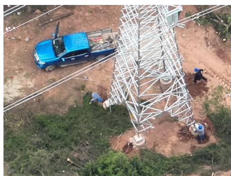
石门 N24 塔基施工场地现状
