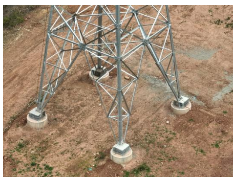
石门 N14 塔基施工场地平整
