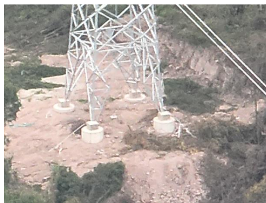
青龙坡 N29 塔基施工场地现状
