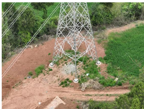
石门 N19 塔基施工场地现状
