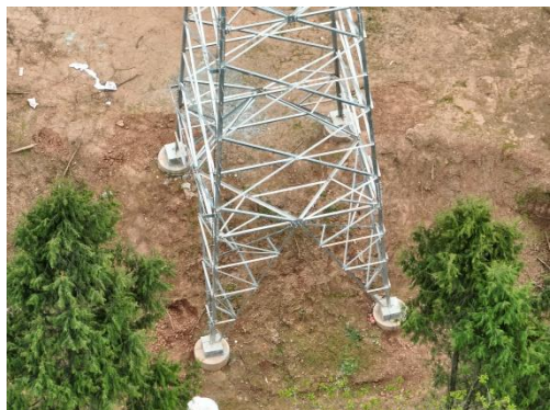
石门 N51 基施工场地现状
