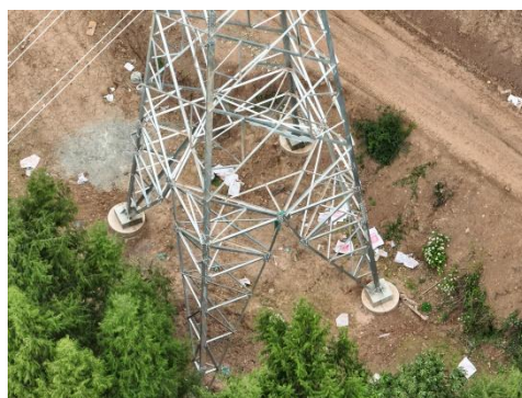
石门 N2 塔基施工场地现状
