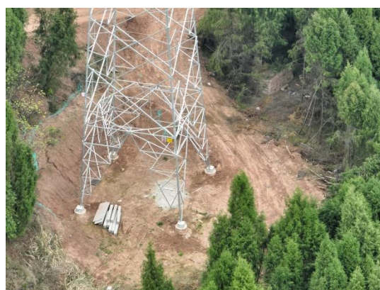
青龙坡 N36 塔基施工场地现状
