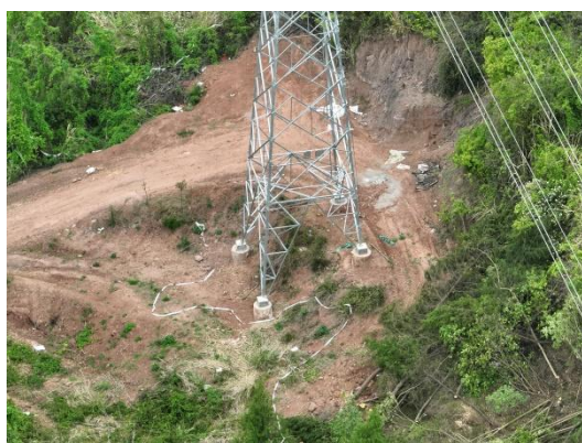
青龙坡 N8 塔基施工场地现状
