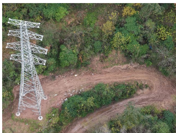
文龙二线 \pi 接线路 N18 塔新修汽运道路未采取临时排水、沉沙、苫盖措施
