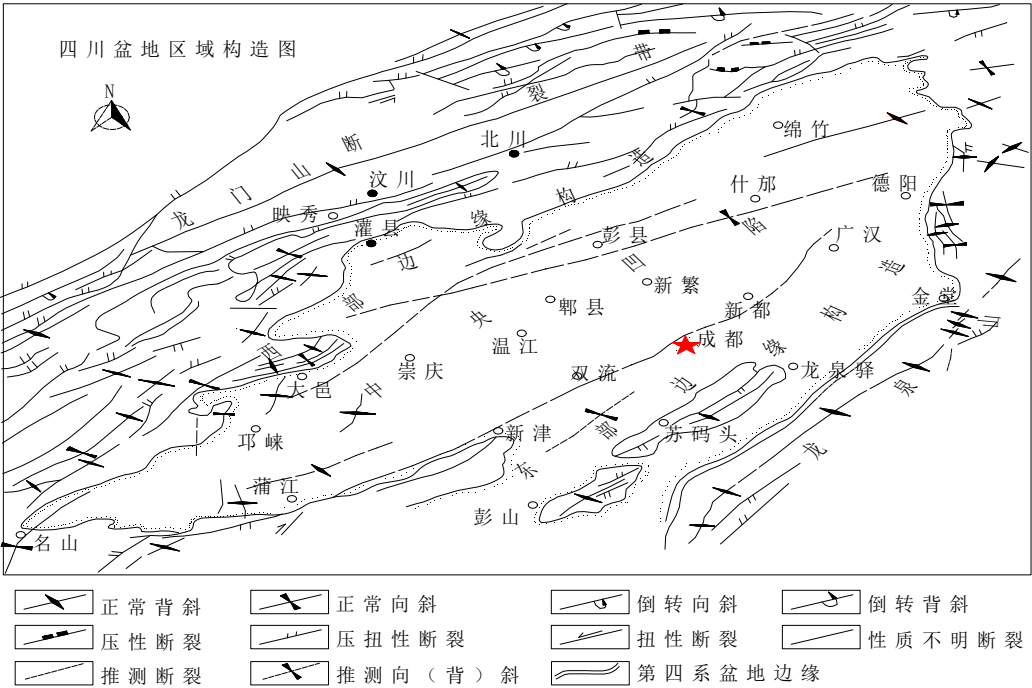
图 1-5 区域构造图
