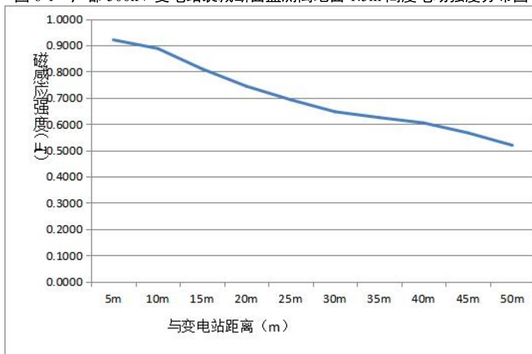
图 6-2 广都 500kV 变电站衰减断面监测离地面 1.5m 高度磁感应强度修正分布图
