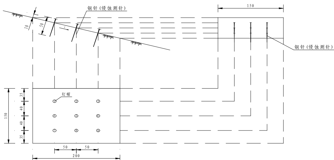
图 3.3.2-1 水土流失简易观测场图
