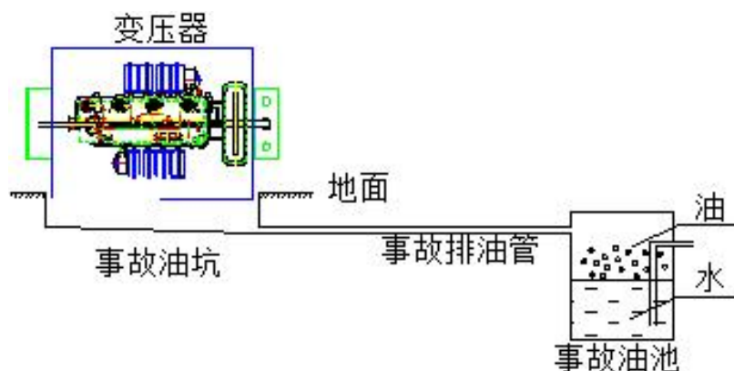
图 6-10 事故油池处理流程示意图
