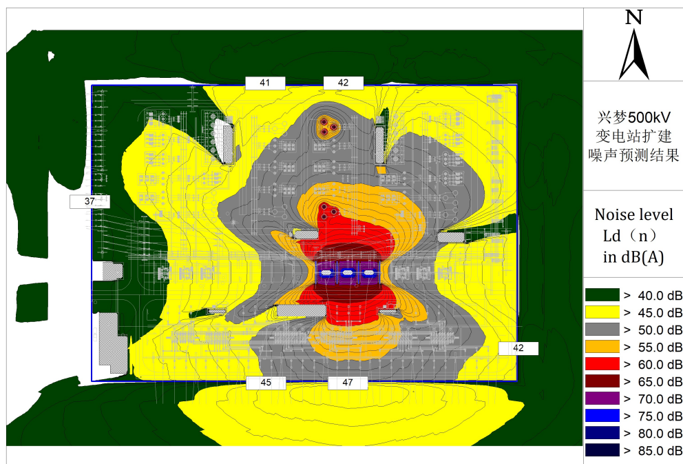
图 6-4 兴梦变电站本次扩建后的噪声预测结果（本期贡献值）
