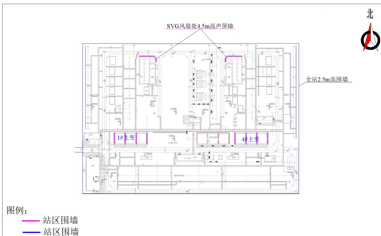
图 6-3 兴梦变电站前期工程已采取的噪声控制措施
