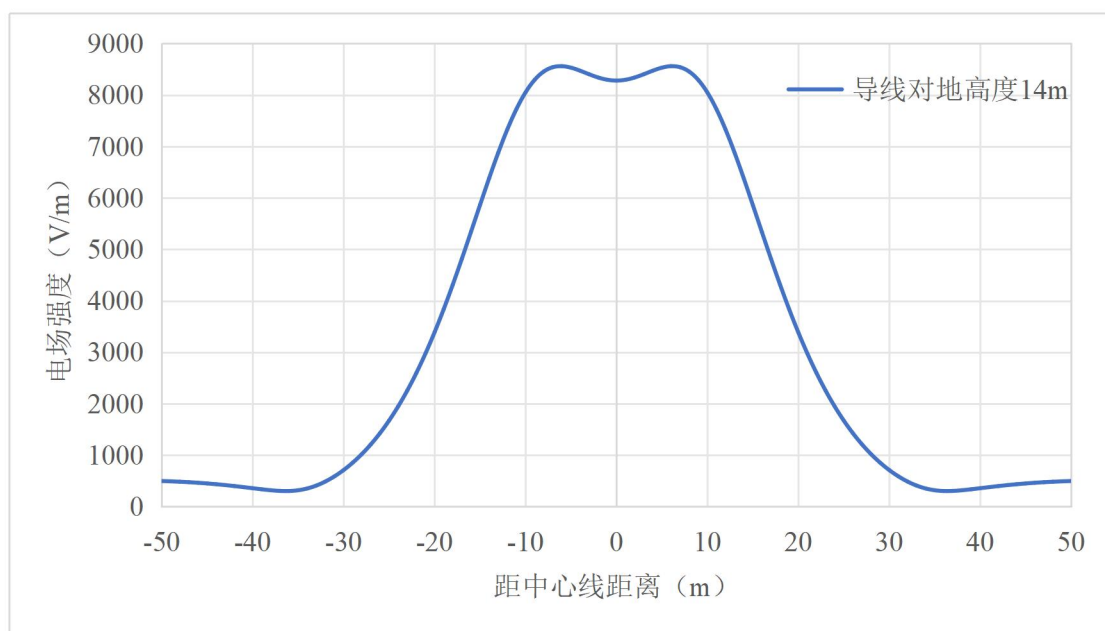
图 6-3 500kV 桃资一二线改造段地面 1.5m 高处工频电场分布曲线
