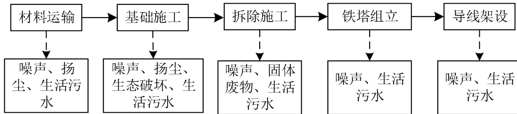
图 3-2 施工期工艺流程及产污环节图
