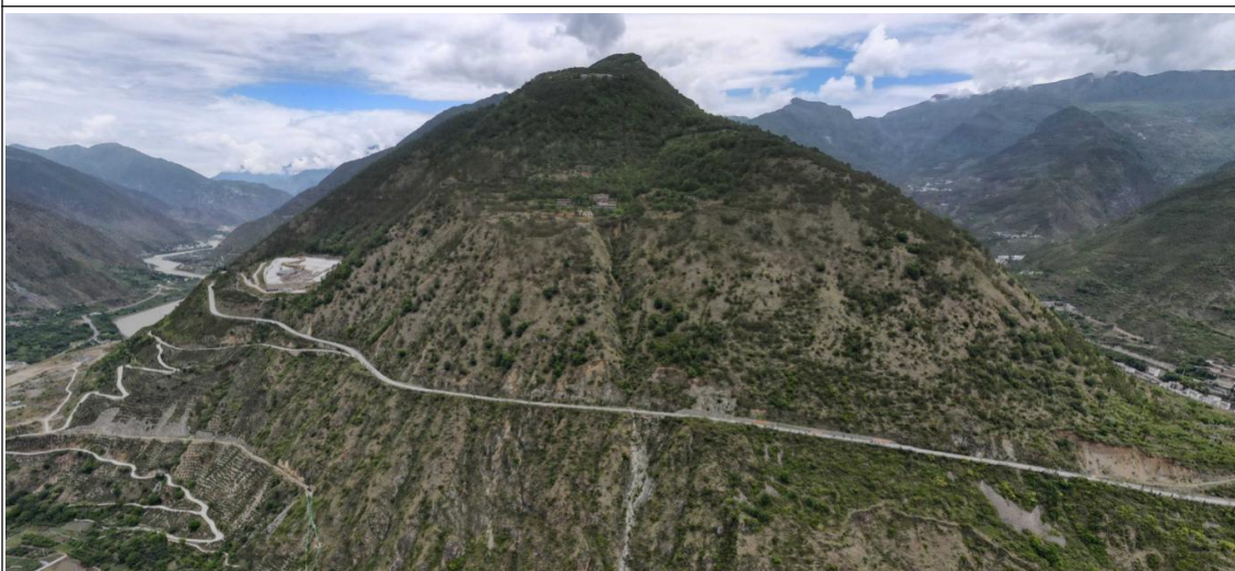
沿线地形地貌
