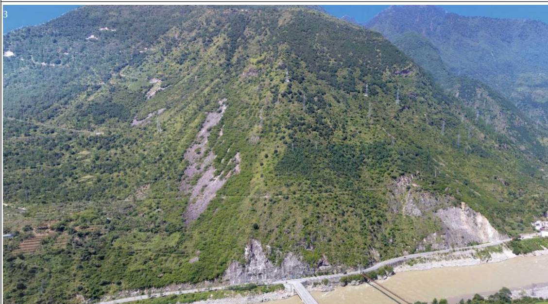
沿线地形地貌
