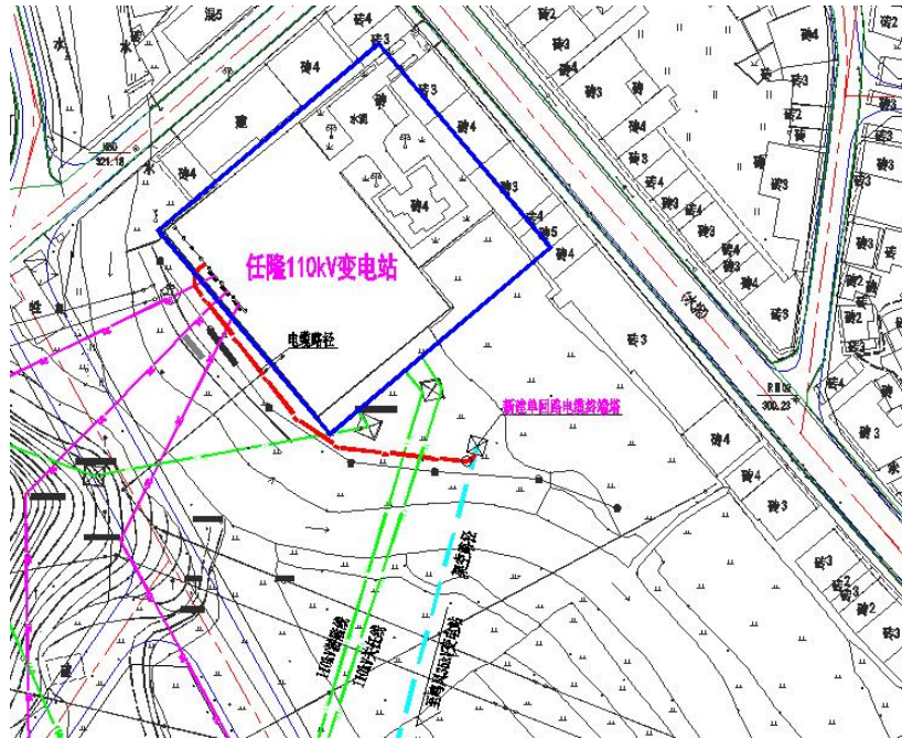
图 2.1-3 任隆 110 千伏变电站出线平面图
