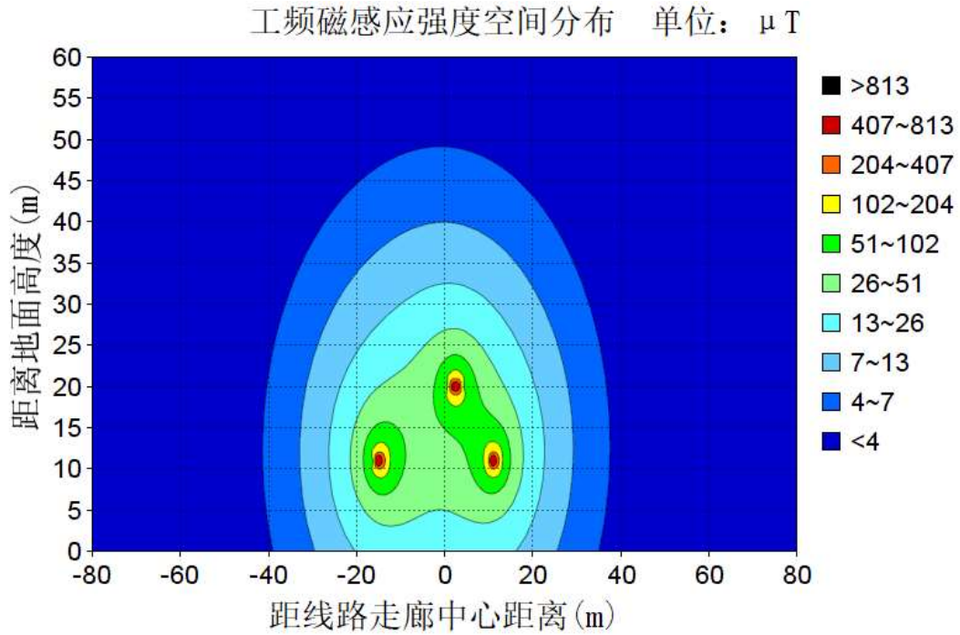
图 6-23 导线对地高度 11m 的磁感应强度等值线图
