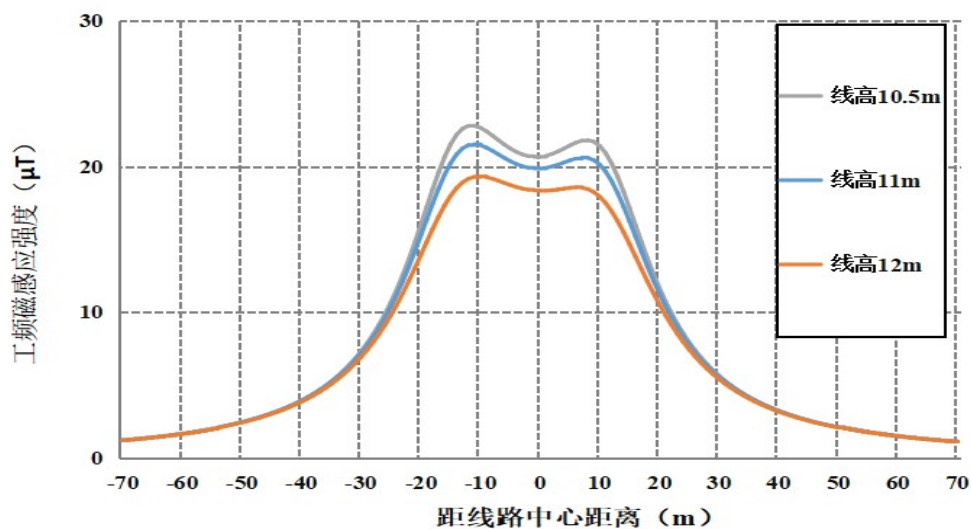
图 6-20 本段线路通过耕地、牧草地等场所最不利塔型磁感应强度随距离变化趋势图
