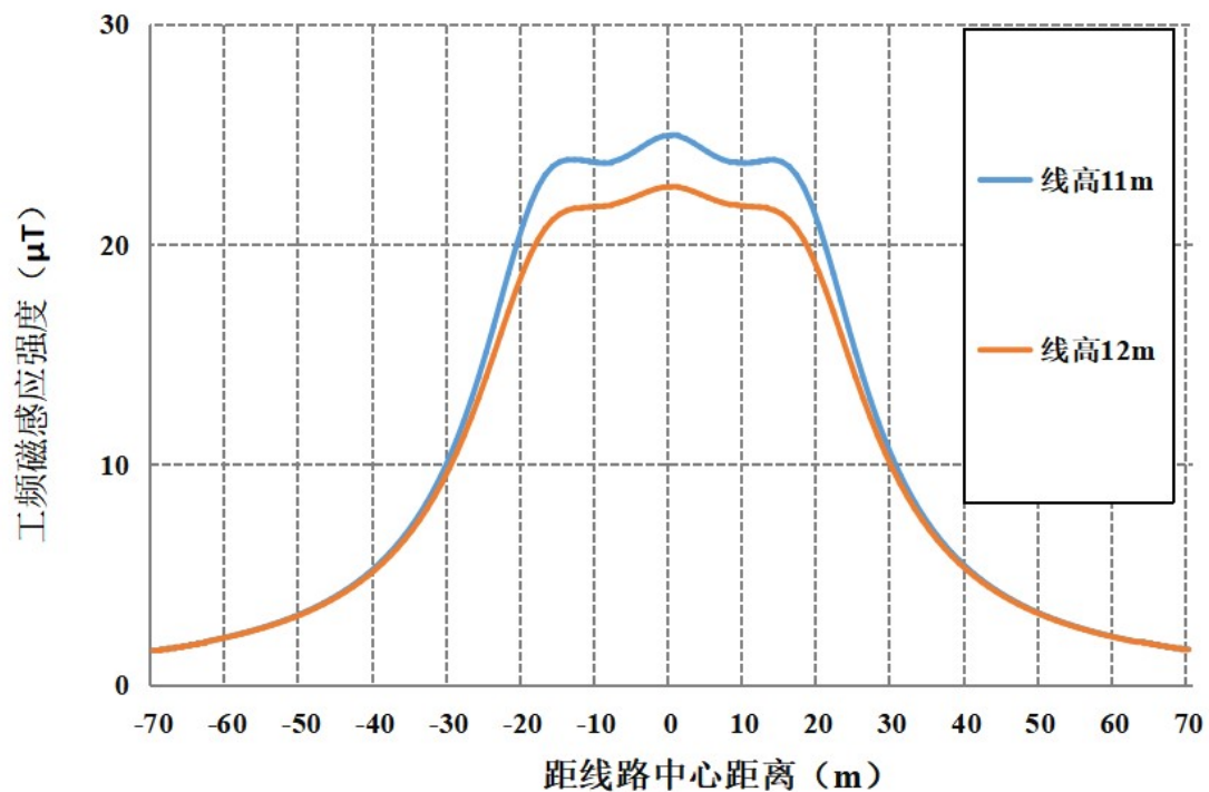
图 6-10 本段线路通过耕地、牧草地等场所最不利塔型磁感应强度随距离变化趋势图
