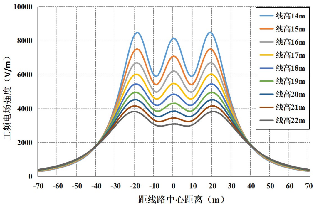
图 6-7 线路在公众曝露区电场强度随距离变化趋势图（距地面 4.5m 高处）
