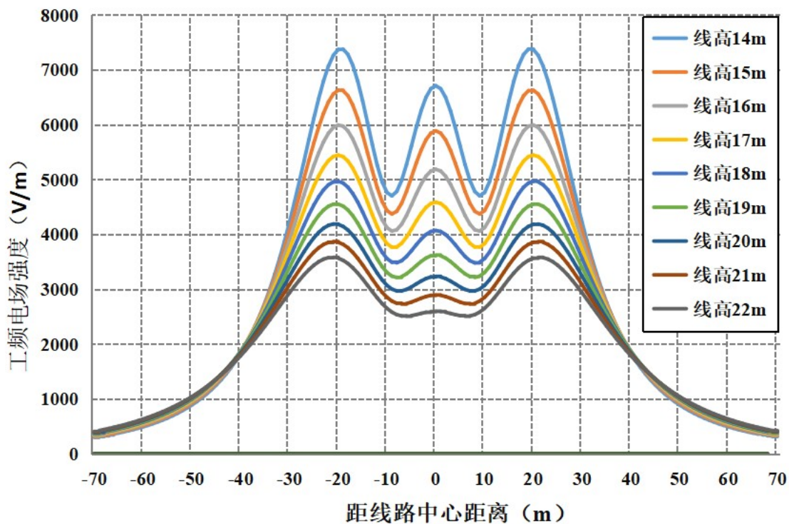
图 6-6 线路在公众曝露区电场强度随距离变化趋势图（距地面 1.5m 高处）
