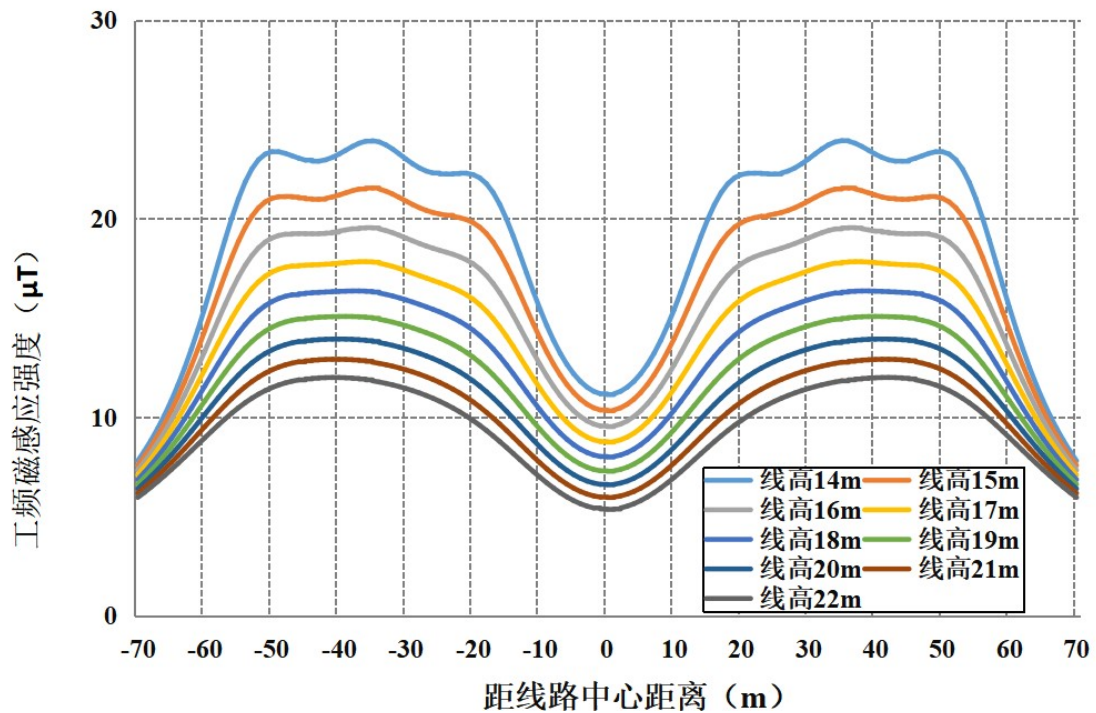
图 6-32 本段线路在民房等公众曝露区域最不利塔型磁感应强度随距离变化趋势图 (离地 4.5m)
