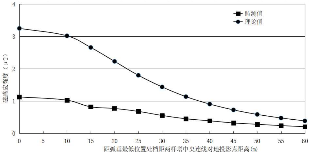
图 6-60 类比线路（瀑布沟电站-东坡一、二回线）磁感应强度随距中心线距变化图
