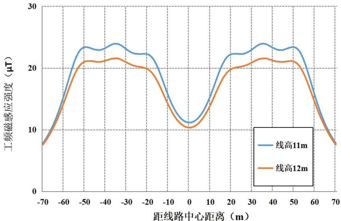
图 6-30 本段线路通过耕地、牧草地等场所最不利塔型磁感应强度随距离变化趋势图
