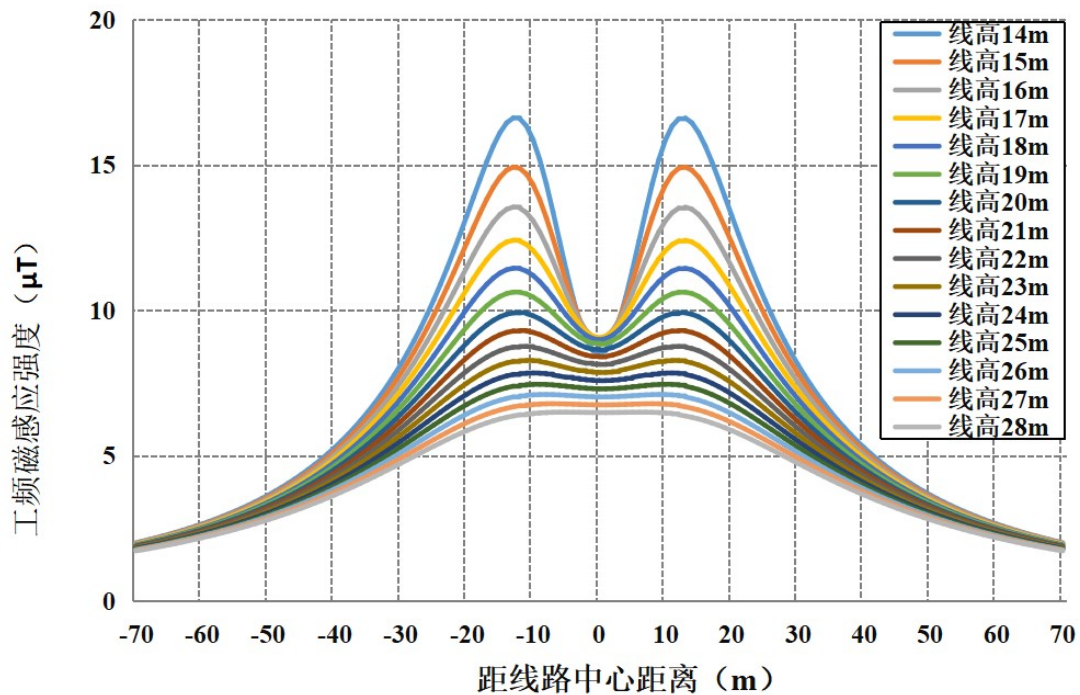
图 6-52 本段线路在民房等公众曝露区域最不利塔型磁感应强度随距离变化趋势图 (离地 4.5m)
