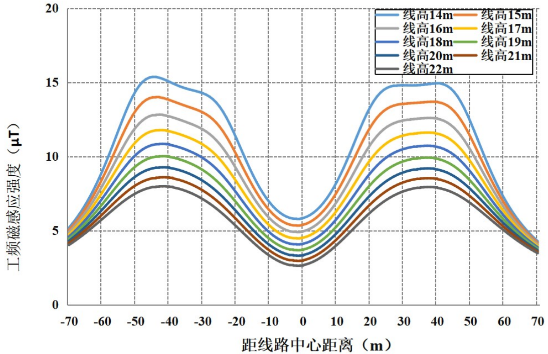
图 6-41 本段线路在民房等公众曝露区域最不利塔型磁感应强度随距离变化趋势图 (离地 1.5m)
