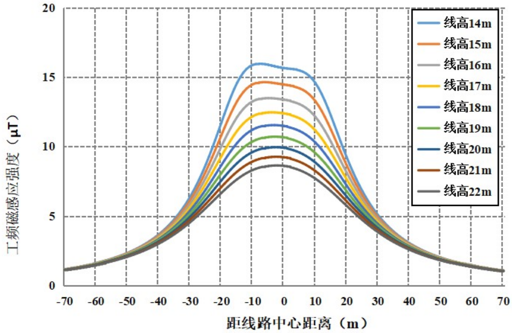
图 6-21 本段线路在民房等公众曝露区域最不利塔型磁感应强度随距离变化趋势图 (离地 1.5m)
