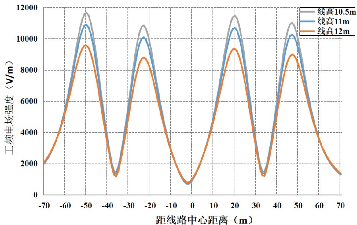
图 6-35 本段线路通过耕地、园地等场所最不利塔型电场强度随距离变化趋势图
