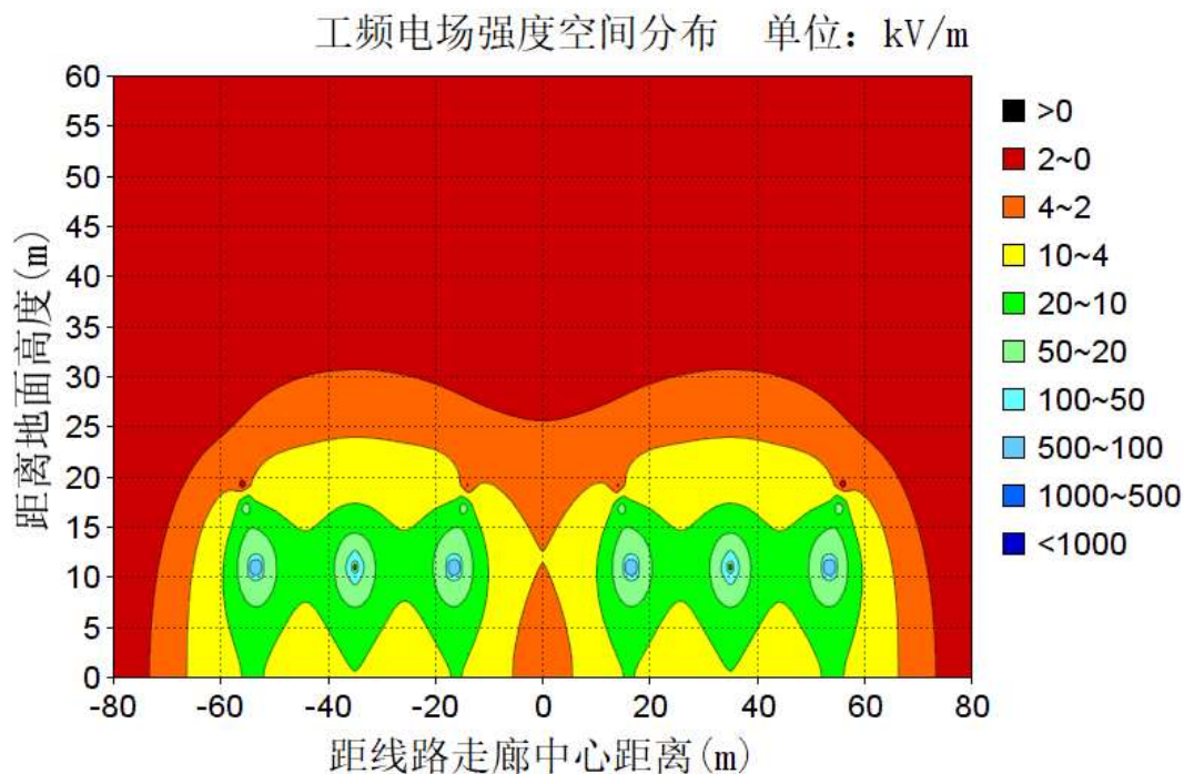
图 6-28 导线对地高度 11m 的电场强度等值线图 (单位: kV/m)
