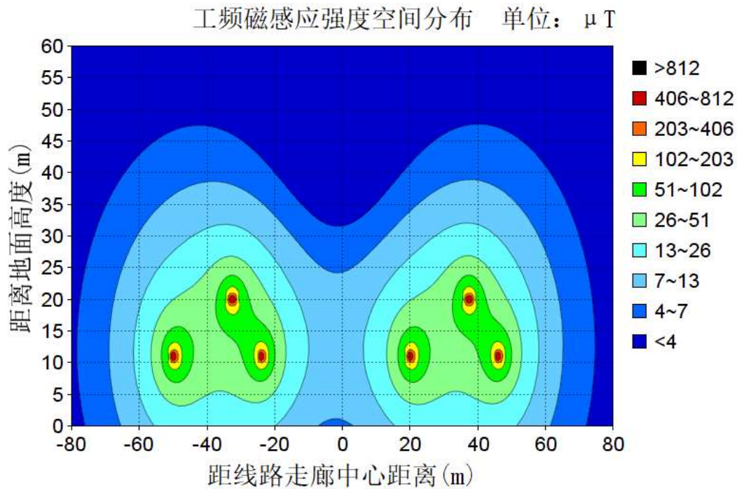
图 6-43 导线对地高度 11m 的磁感应强度等值线图
