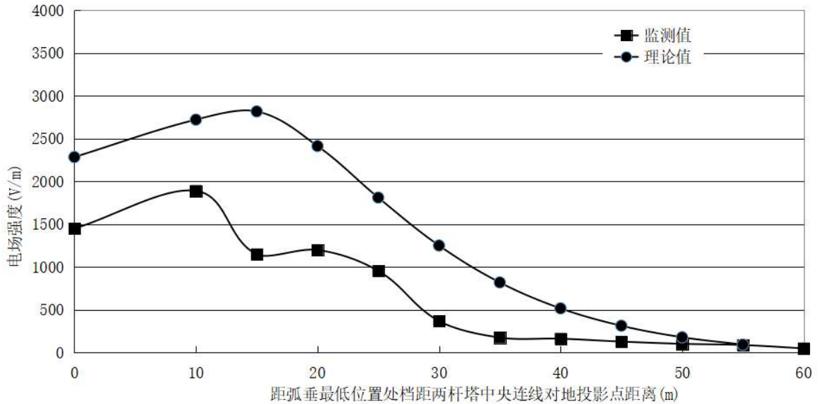
图 6-59 类比线路（瀑布沟电站-东坡一、二回线）电场强度随距中心线距变化趋势图
