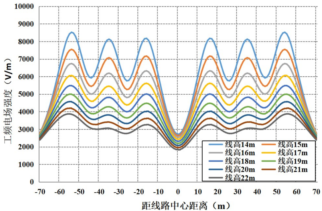
图 6-27 线路在公众曝露区电场强度随距离变化趋势图（距地面 4.5m 高处）
