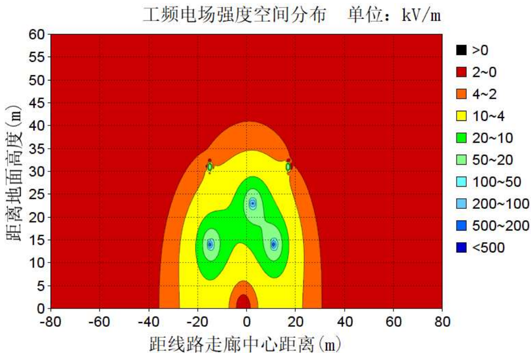
图 6-19 导线对地高度 14m 的电场强度等值线图 (单位: kV/m)
