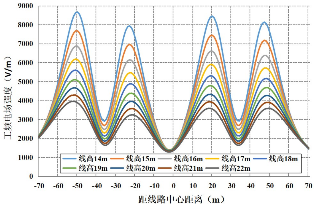
图 6-37 线路在公众曝露区电场强度随距离变化趋势图（距地面 4.5m 高处）
