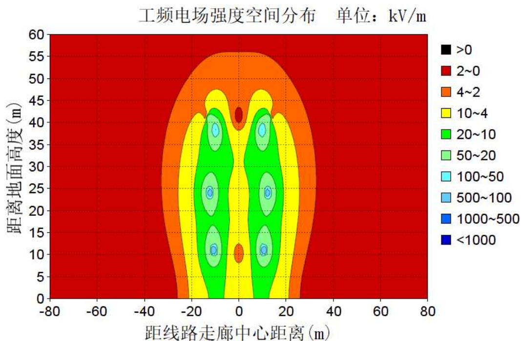
图 6-48 导线对地高度 11m 的电场强度等值线图 (单位: kV/m)
