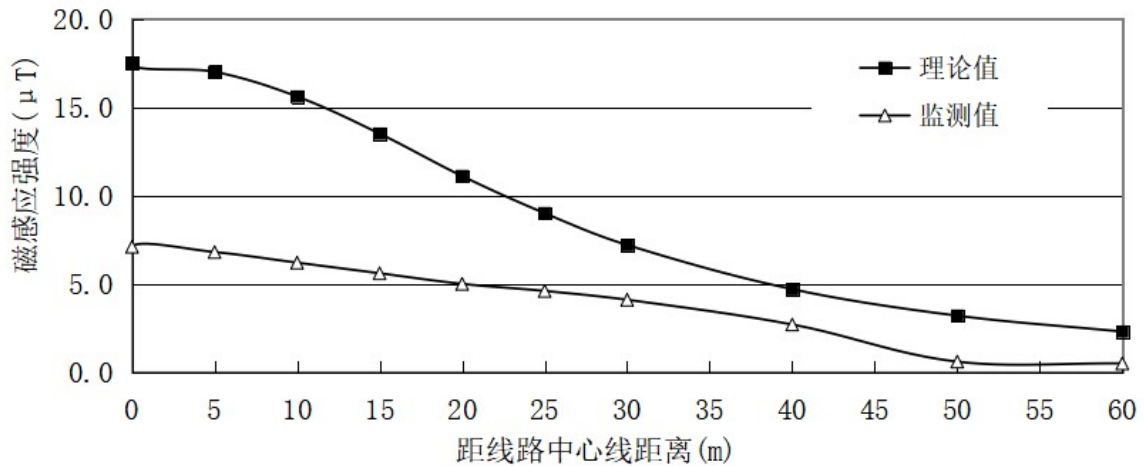
图 6-56 类比线路（500kV 洪板一线）磁感应强度随距中心线距离变化趋势图
