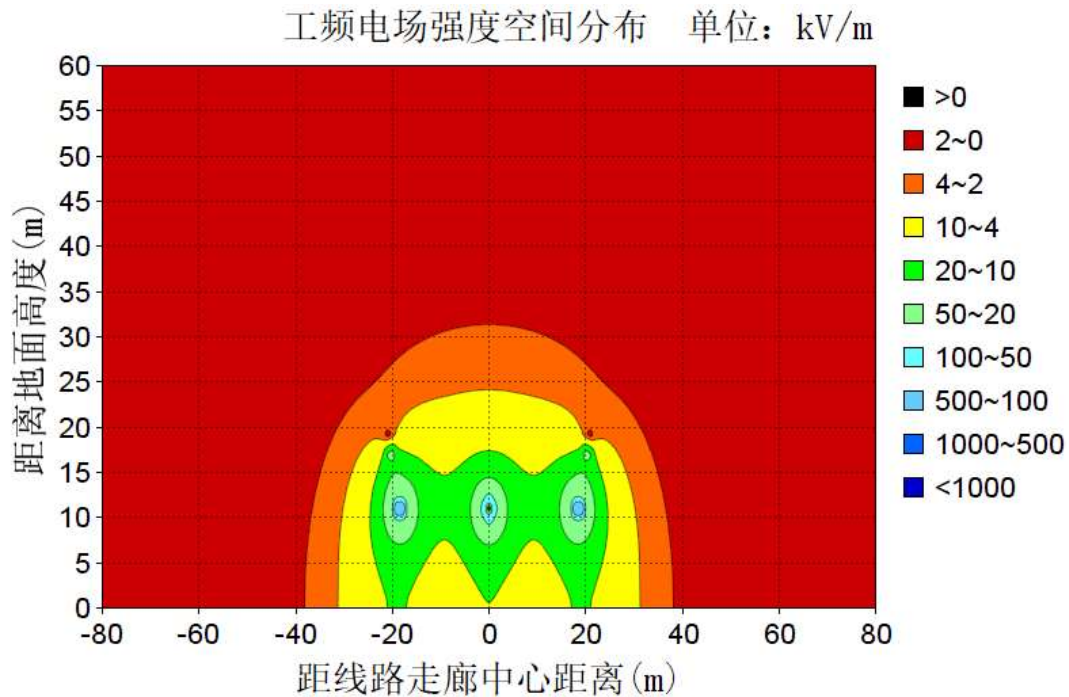
图 6-8 导线对地高度 11m 的电场强度等值线图 (单位: kV/m)
