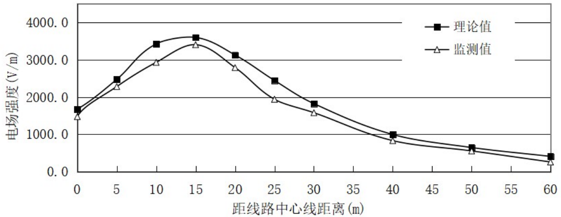
图 6-57 类比线路（500kV 洪板二线）电场强度随距中心线距变化趋势图
