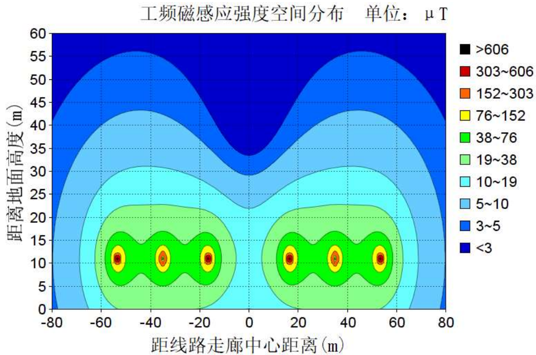
图 6-33 导线对地高度 11m 的磁感应强度等值线图
