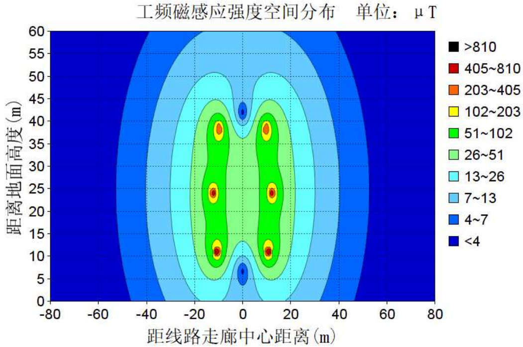
图 6-53 导线对地高度 11m 的磁感应强度等值线图
