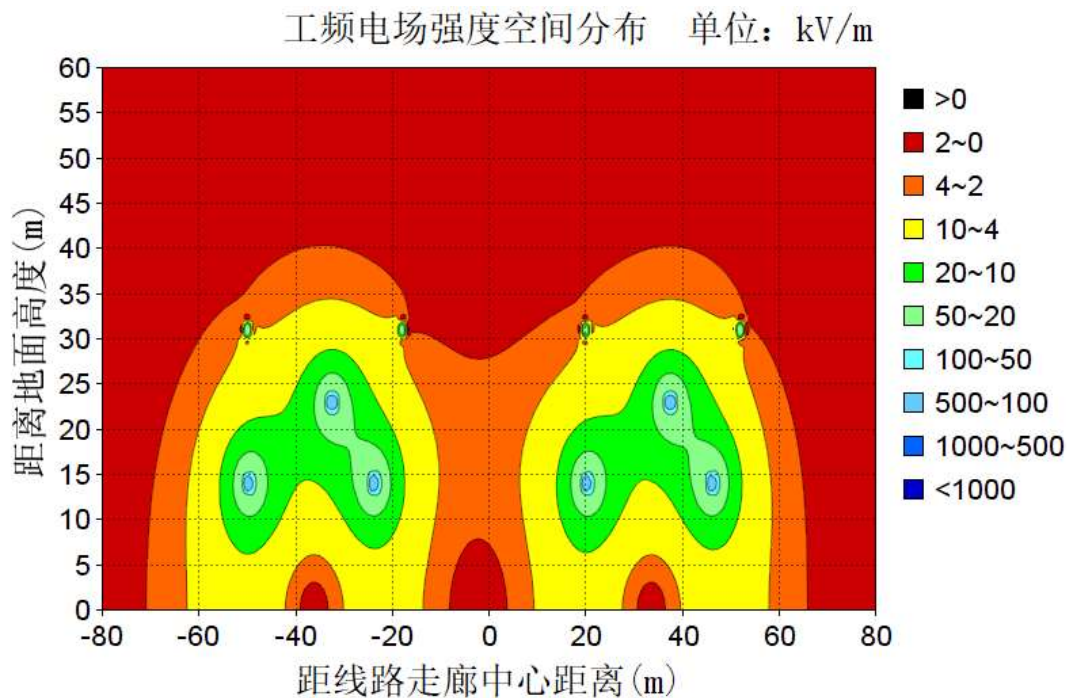
图 6-39 导线对地高度 14m 的电场强度等值线图 (单位: kV/m)
