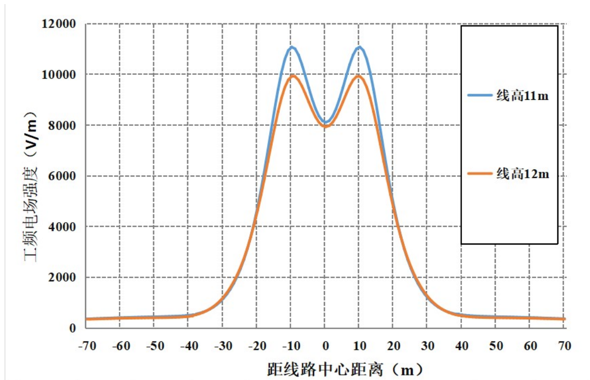
图 6-45 本段线路通过耕地、园地等场所最不利塔型电场强度随距离变化趋势图
