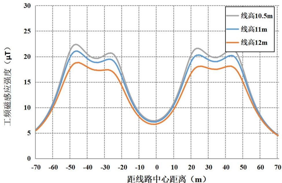
图 6-40 本段线路通过耕地、牧草地等场所最不利塔型磁感应强度随距离变化趋势图
