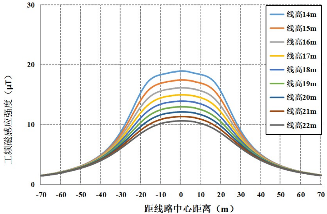
图 6-11 本段线路在民房等公众曝露区域最不利塔型磁感应强度随距离变化趋势图 (离地 1.5m)
