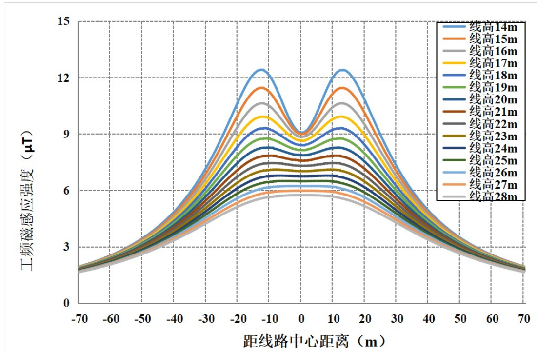
图 6-51 本段线路在民房等公众曝露区域最不利塔型磁感应强度随距离变化趋势图 (离地 1.5m)
