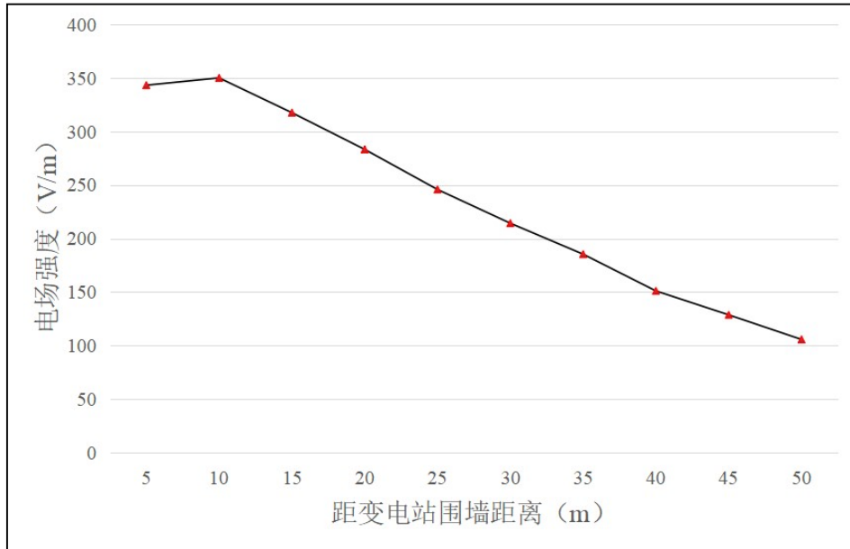
图 6-1 类比变电站围墙外电场强度随距离变化趋势图
