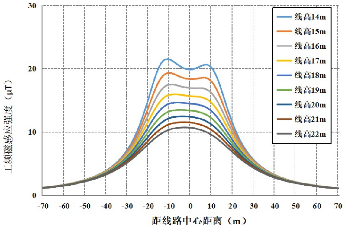
图 6-22 本段线路在民房等公众曝露区域最不利塔型磁感应强度随距离变化趋势图 (离地 4.5m)
