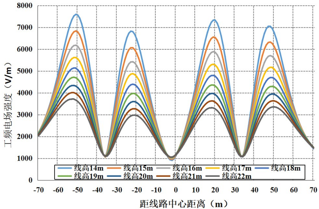
图 6-36 线路在公众曝露区电场强度随距离变化趋势图（距地面 1.5m 高处）
