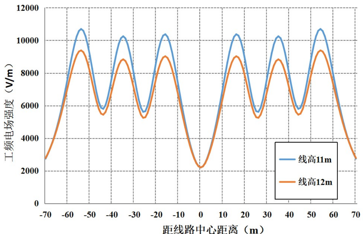
图 6-25 本段线路通过耕地、园地等场所最不利塔型电场强度随距离变化趋势图
