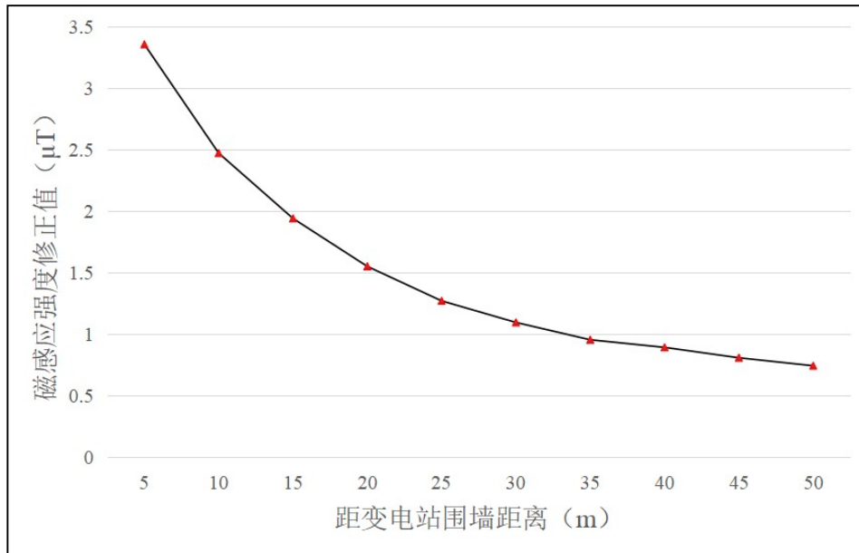
图 6-2 类比变电站围墙外磁感应强度随距离变化趋势图
