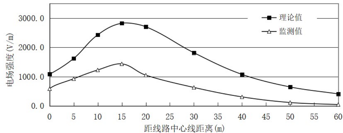
图 6-55 类比线路（500kV 洪板一线）电场强度随距中心线距离变化趋势图
