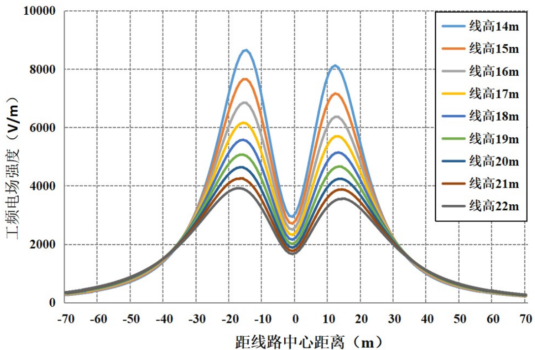
图 6-17 线路在公众曝露区电场强度随距离变化趋势图（距地面 4.5m 高处）
