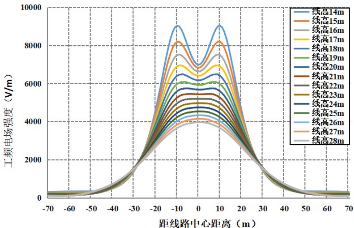
图 6-47 线路在公众曝露区电场强度随距离变化趋势图（距地面 4.5m 高处）
