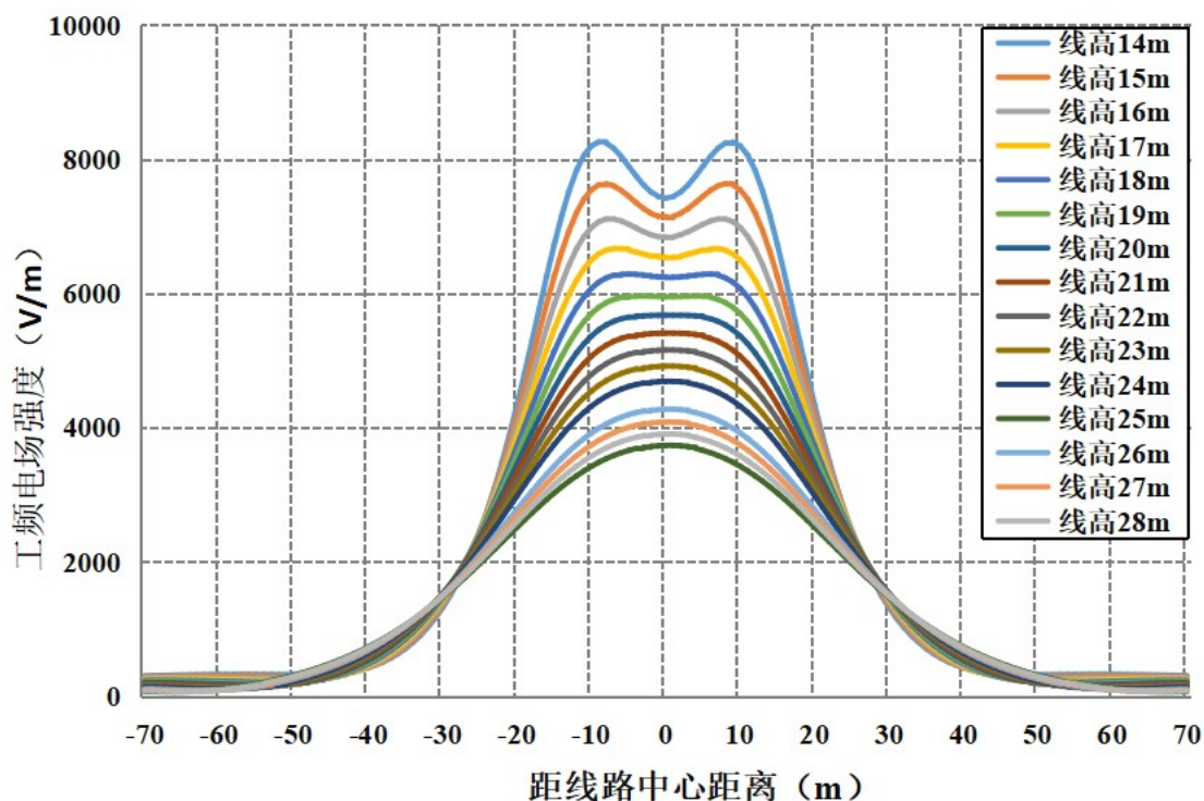
图 6-46 线路在公众曝露区电场强度随距离变化趋势图（距地面 1.5m 高处）
