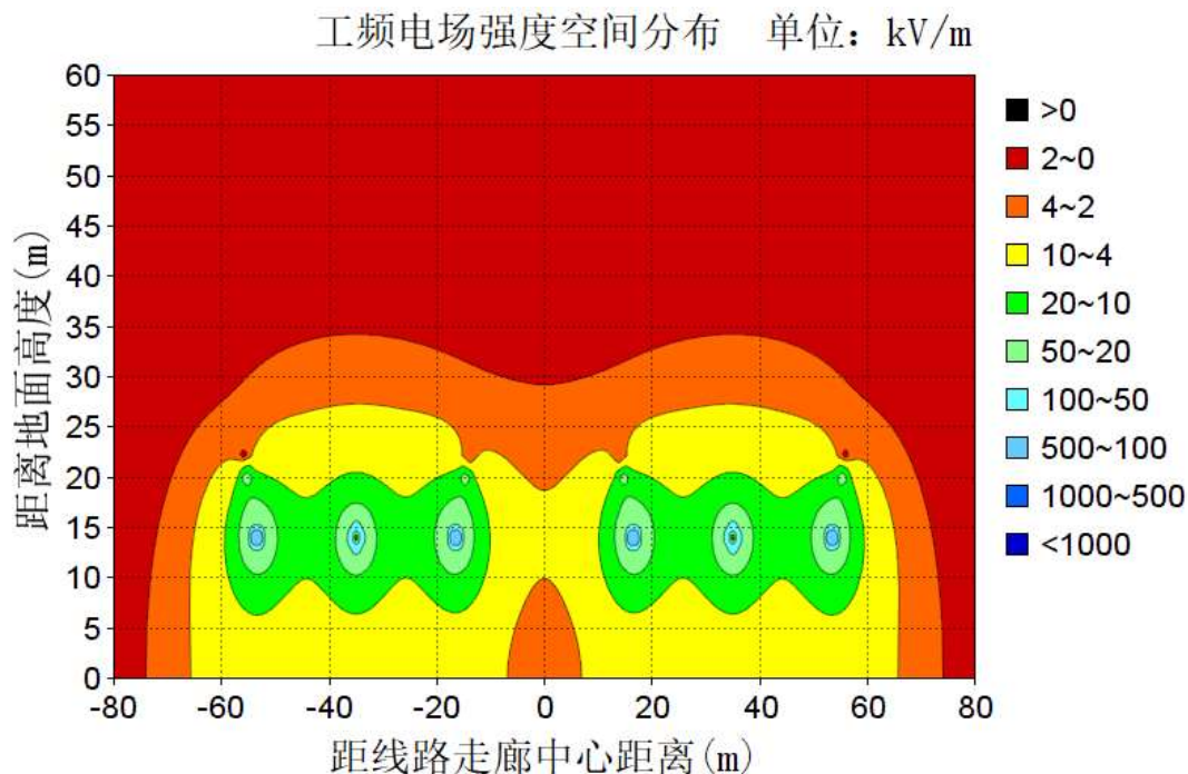
图 6-29 导线对地高度 14m 的电场强度等值线图 (单位: kV/m)
