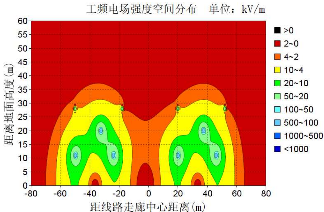
图 6-38 导线对地高度 11m 的电场强度等值线图 (单位: kV/m)
