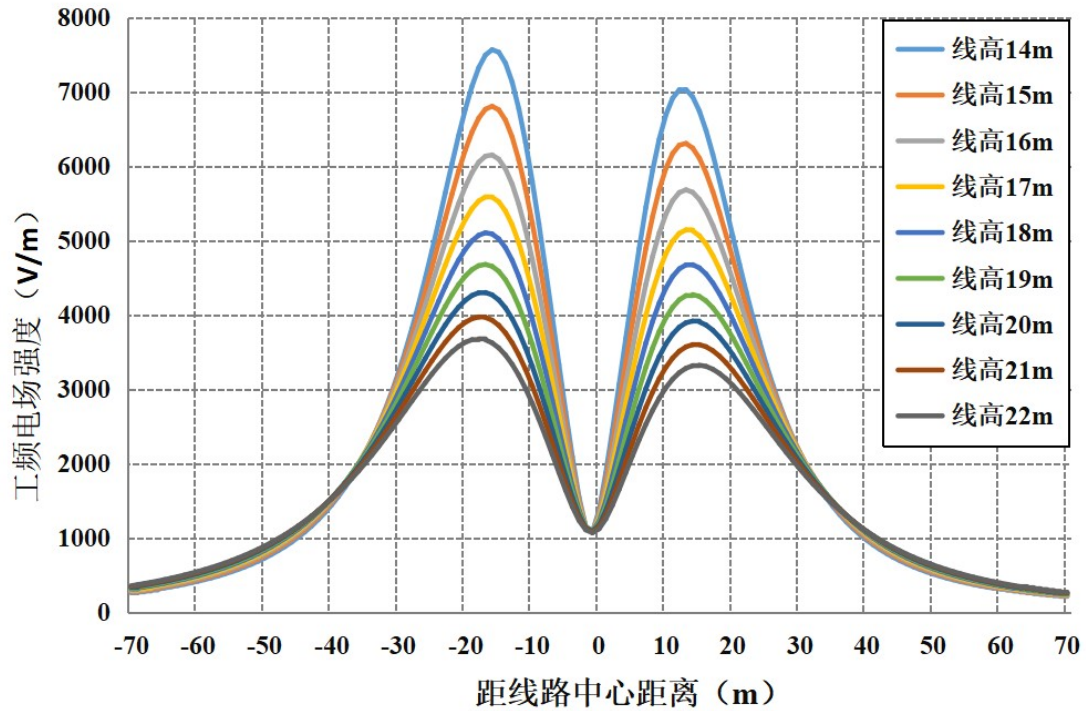
图 6-16 线路在公众曝露区电场强度随距离变化趋势图（距地面 1.5m 高处）
