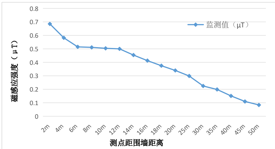
图 6-4 丹景 500kV 变电站衰减断面监测离地面 1.5m 高度磁感应强度分布图
