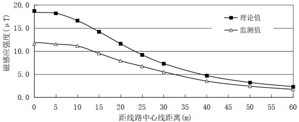
图 6-58 类比线路（500kV 洪板二线）磁感应强度随距中心线距变化图
