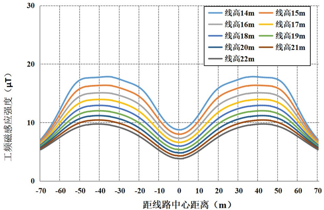
图 6-31 本段线路在民房等公众曝露区域最不利塔型磁感应强度随距离变化趋势图 (离地 1.5m)
