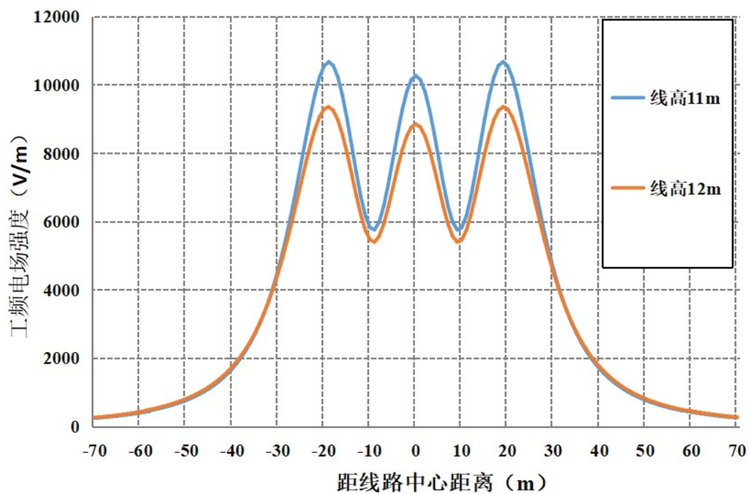
图 6-5 本段线路通过耕地、园地等场所最不利塔型电场强度随距离变化趋势图
