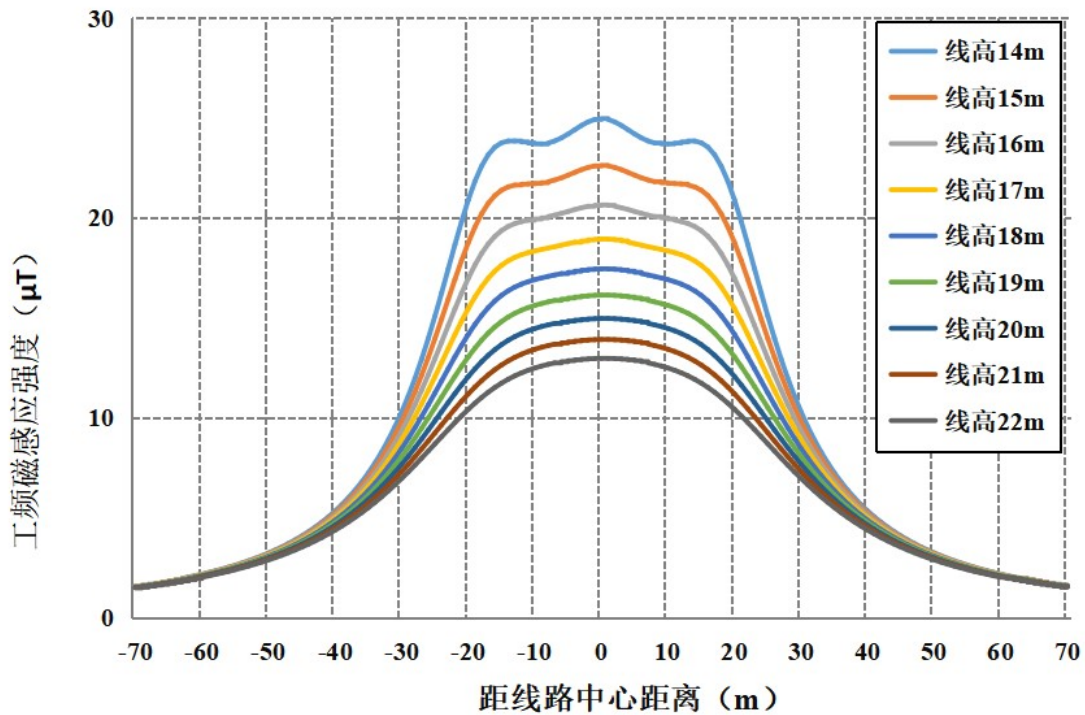
图 6-12 本段线路在民房等公众曝露区域最不利塔型磁感应强度随距离变化趋势图 (离地 4.5m)
