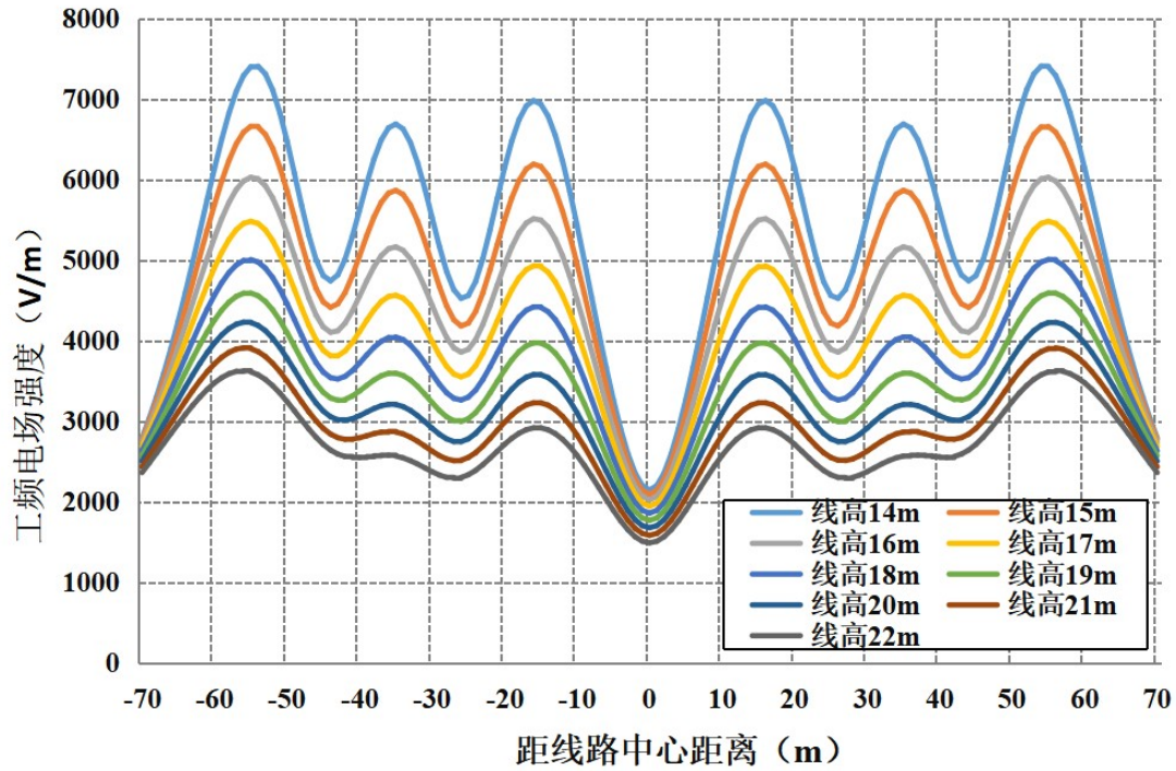
图 6-26 线路在公众曝露区电场强度随距离变化趋势图（距地面 1.5m 高处）
