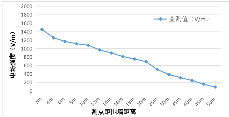
图 6-3 丹景 500kV 变电站衰减断面监测离地面 1.5m 高度电场强度分布图
