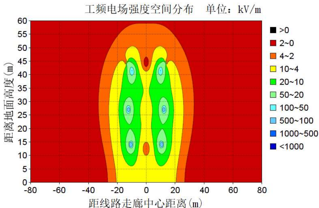
图 6-49 导线对地高度 14m 的电场强度等值线图 (单位: kV/m)
