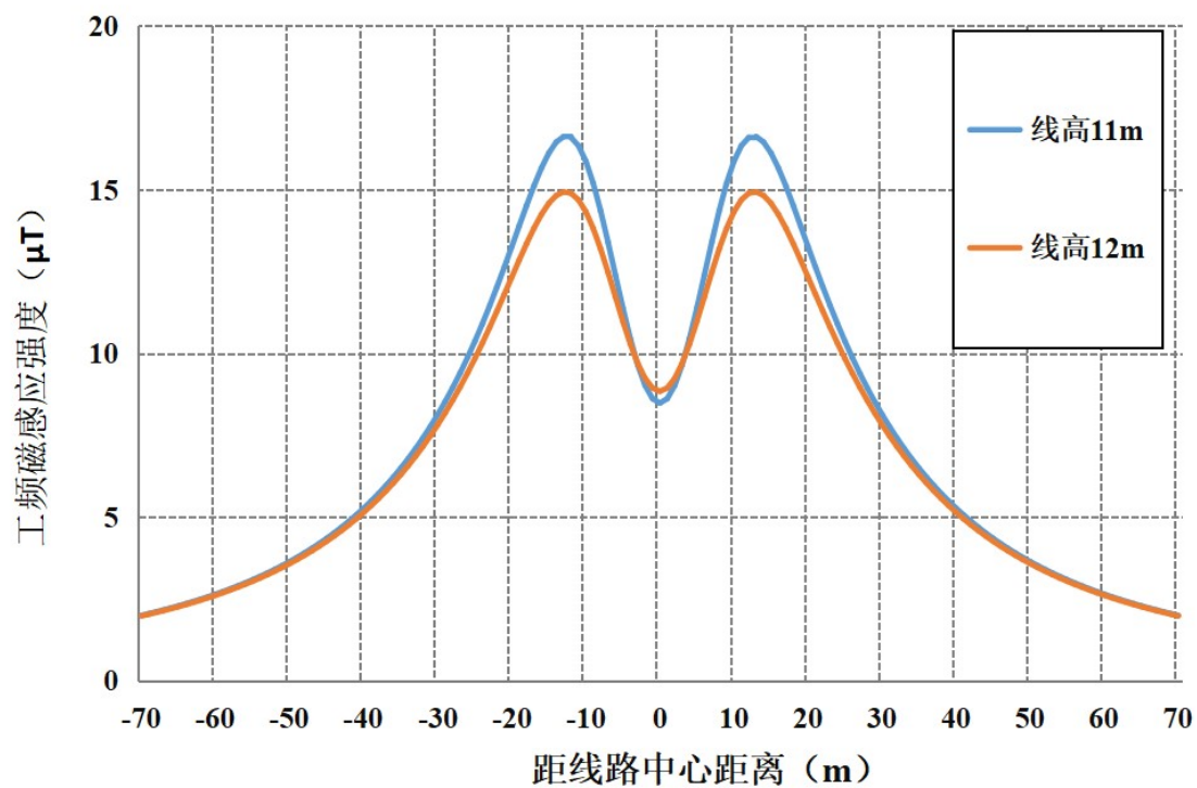
图 6-50 本段线路通过耕地、牧草地等场所最不利塔型磁感应强度随距离变化趋势图
