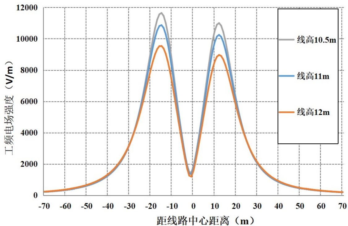
图 6-15 本段线路通过耕地、园地等场所最不利塔型电场强度随距离变化趋势图
