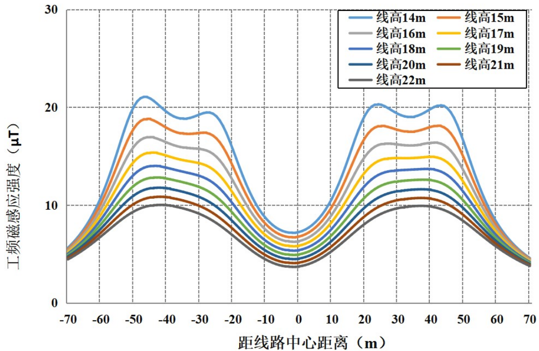
图 6-42 本段线路在民房等公众曝露区域最不利塔型磁感应强度随距离变化趋势图 (离地 4.5m)
