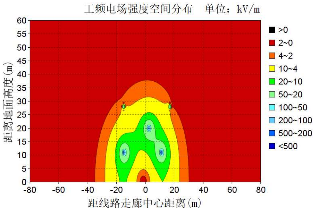
图 6-18 导线对地高度 11m 的电场强度等值线图 (单位: kV/m)
