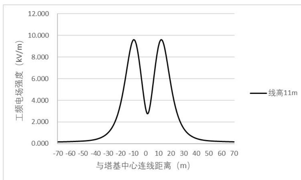
图 6-1 双回段线路在通过耕作、畜牧养殖及道路等区域电场强度随距离变化趋势图
