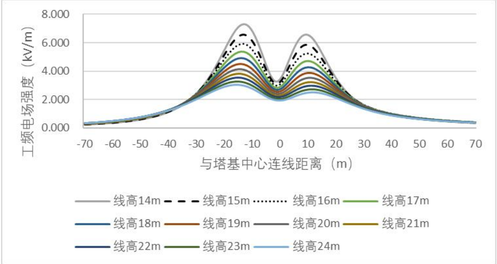
图 6-11 单回路线路在通过公众曝露区电场强度随距离变化趋势图（离地 1.5m 高处）
