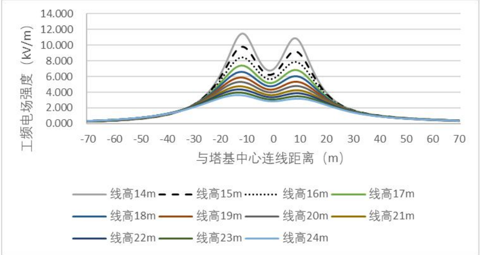
图 6-13 单回段线路在通过公众曝露区电场强度随距离变化趋势图（离地 7.5m 高处）
