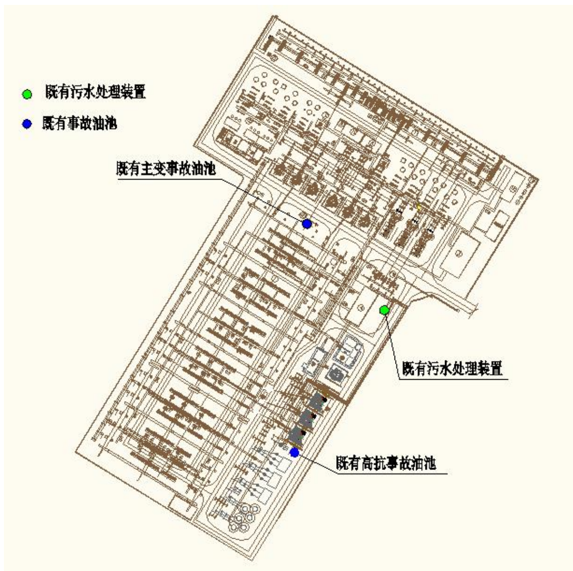
图 3-1 月城变电站前期工程主要环保设施布置图
