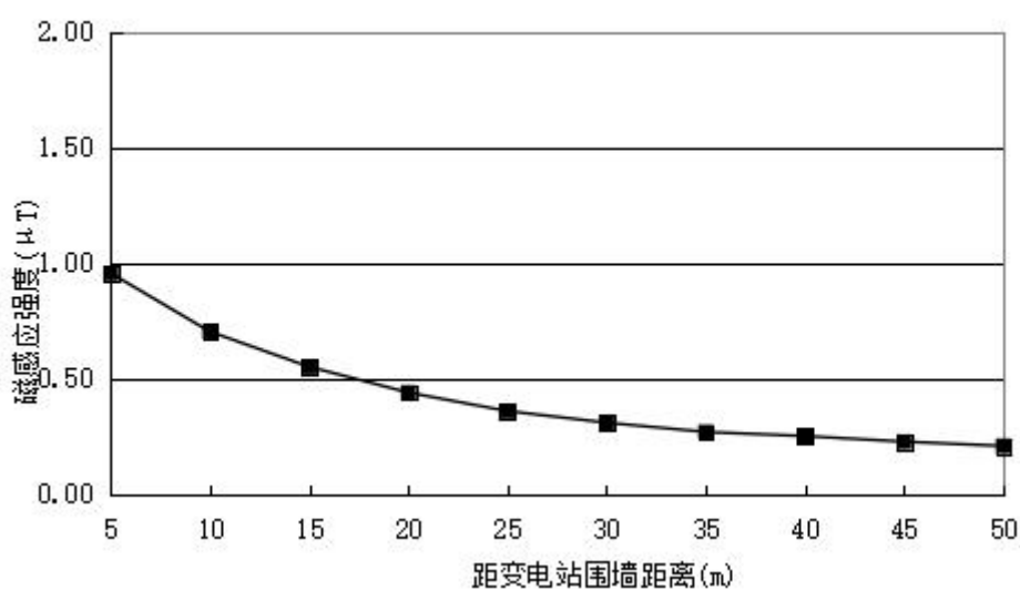
图 6-2 变电站南侧衰减断面监测离地面 1.5m 高度磁感应强度修正分布图
