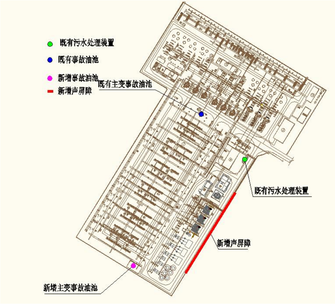
图 3-4 变电站本次扩建后环保措施布置图
