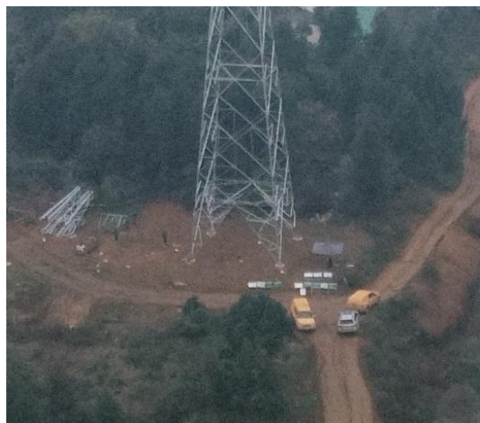
N3 塔位及施工道路
