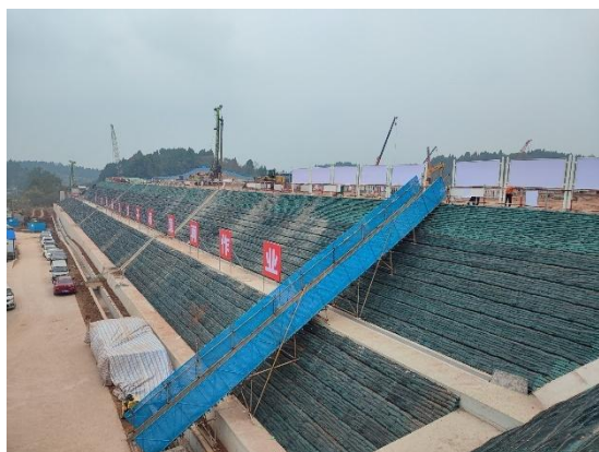
图8-7 变电站生态护坡
