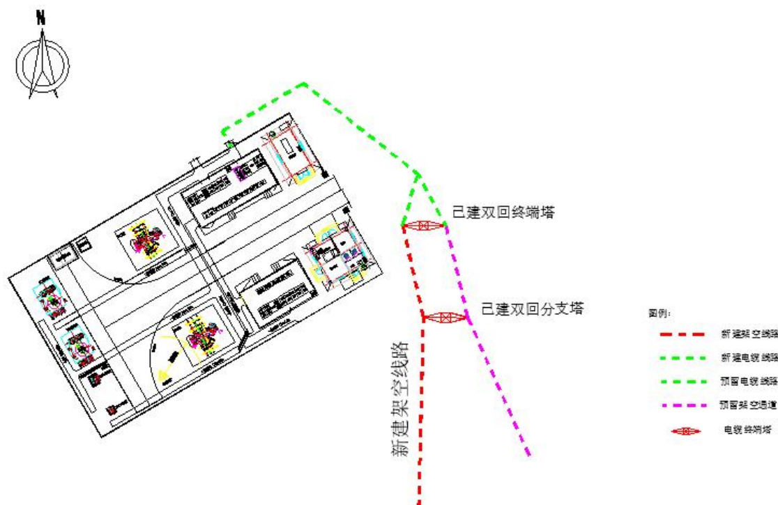
图 2.1-3 林庆站 35kV 出线示意图
