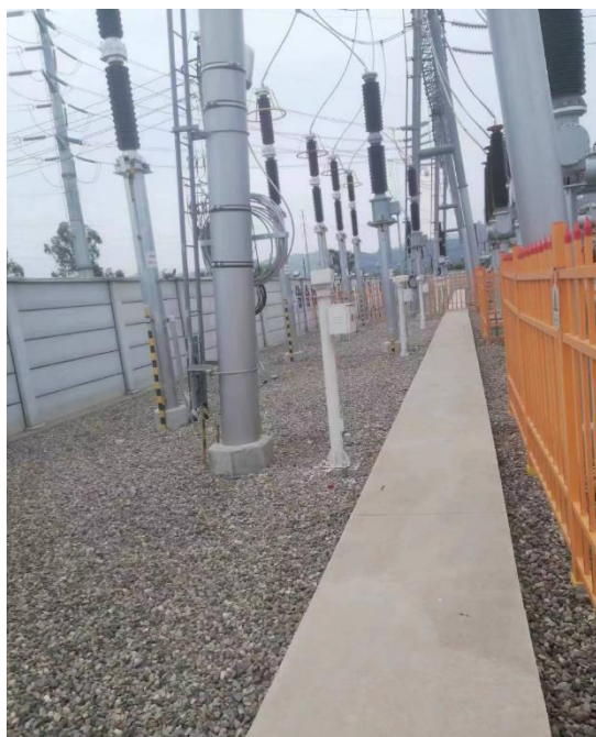
红砂220kv变电站间隔扩建处设置碎石压盖
