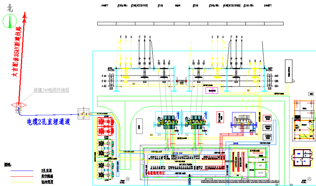
图 2-1 110kV 太吉站出线示意图
