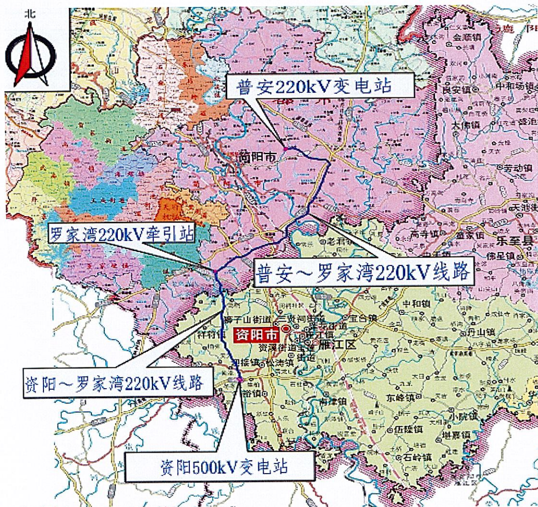
图 1.1-1 本工程地理位置及路径图
