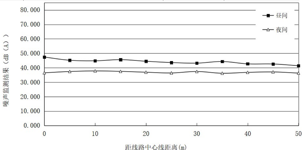
图 6-9 类比线路（500kV 雅安~尖山双回线路）噪声度随距中心线距离变化趋势图
