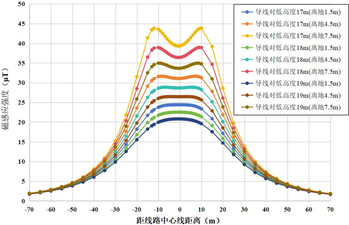
(续) 图 6-4 本段线路在民房等公众曝露区域最不利塔型磁感应强度随距离变化趋势图
