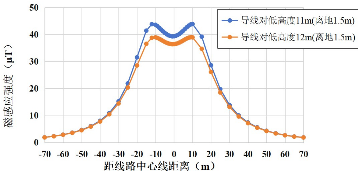
图 6-3 本段线路通过耕地、牧草地等场所最不利塔型磁感应强度随距离变化趋势图
