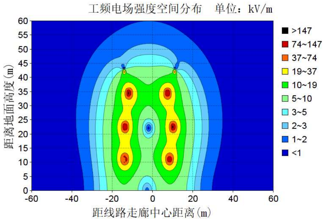
图 6-5 不同高度处电场强度等值线图（导线对地高度 11m） 工频电场强度空间分布 单位: kV/m
