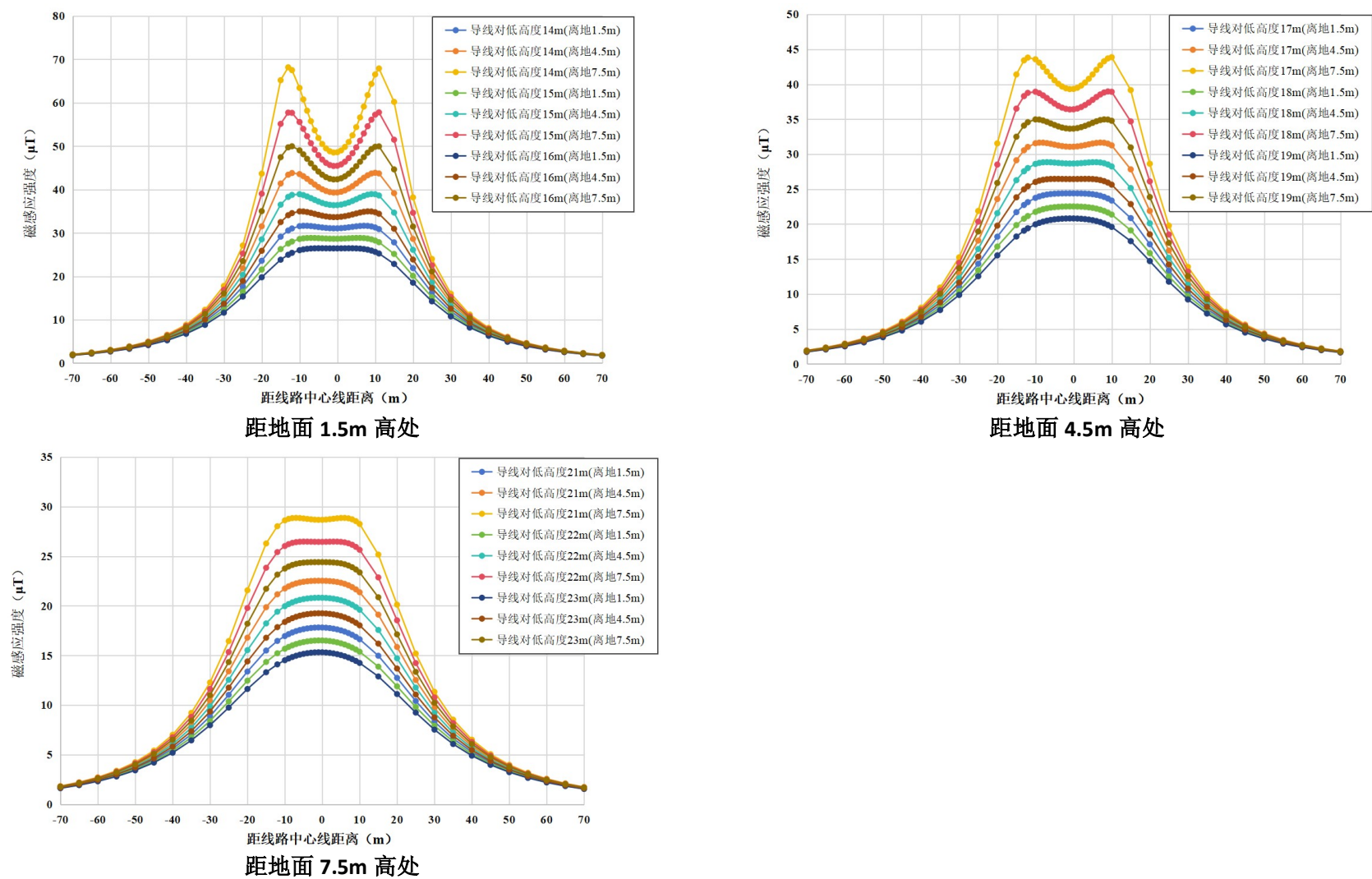
图 6-2 线路在公众曝露区电场强度随距离变化趋势图
