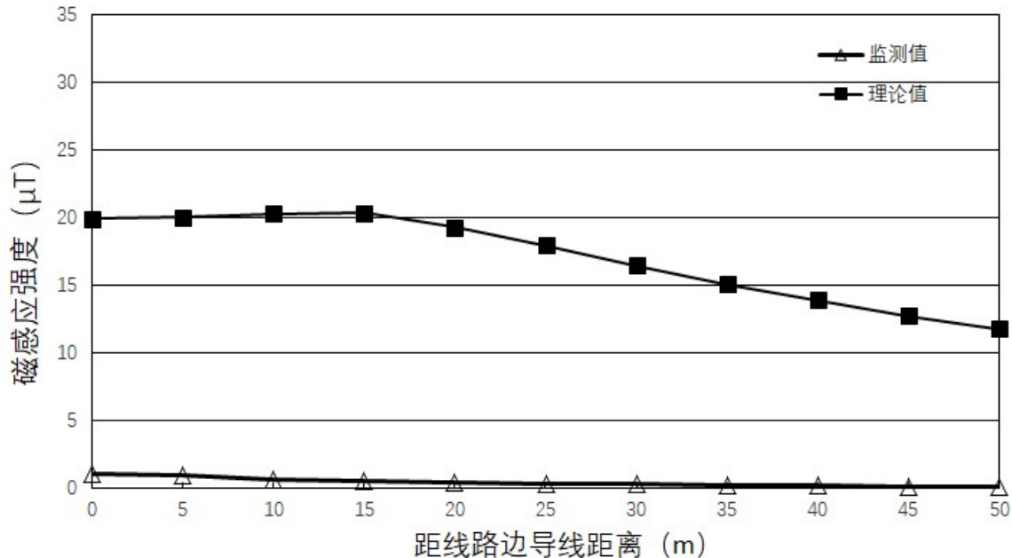
图 6-8 类比线路（梦山一二线）磁感应强度随距中心线距离变化趋势图
