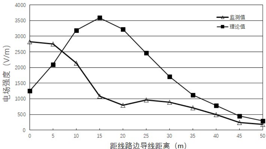
图 6-7 类比线路（梦山一二线）电场强度随距中心线距离变化趋势图
