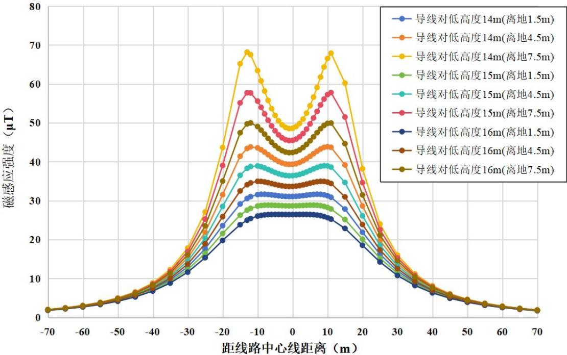
图 6-4 本段线路在民房等公众暴露区域最不利塔型磁感应强度随距离变化趋势图
