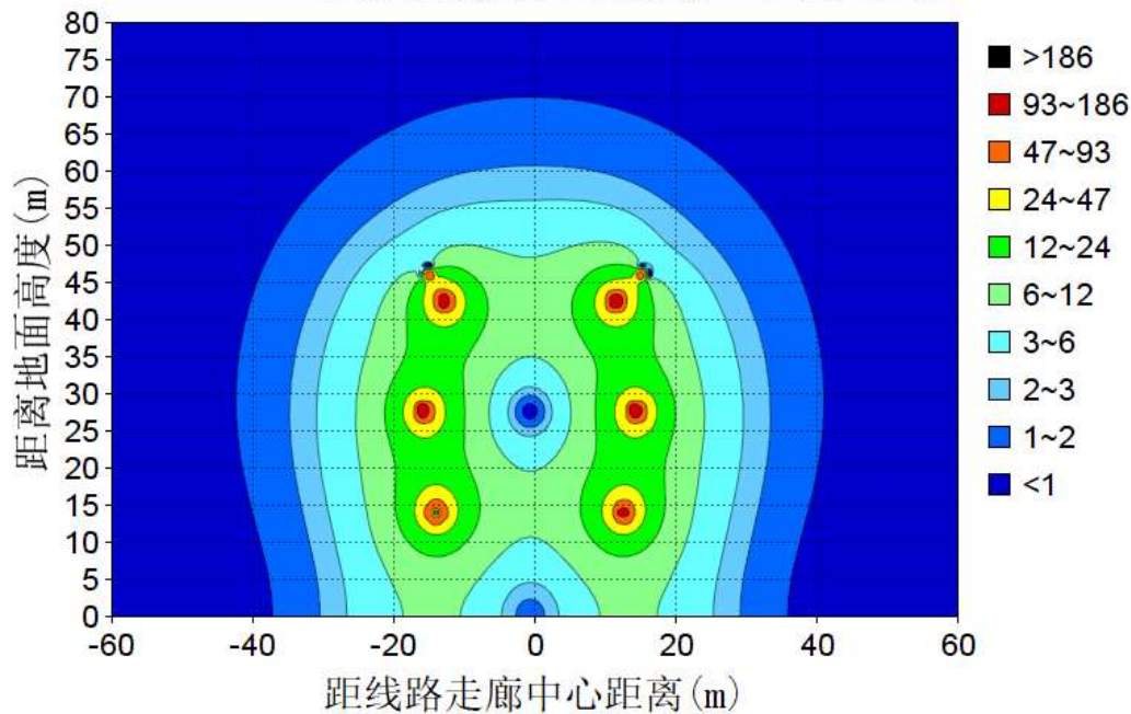
图 6-6 不同高度处电场强度等值线图（导线对地高度 14m）
