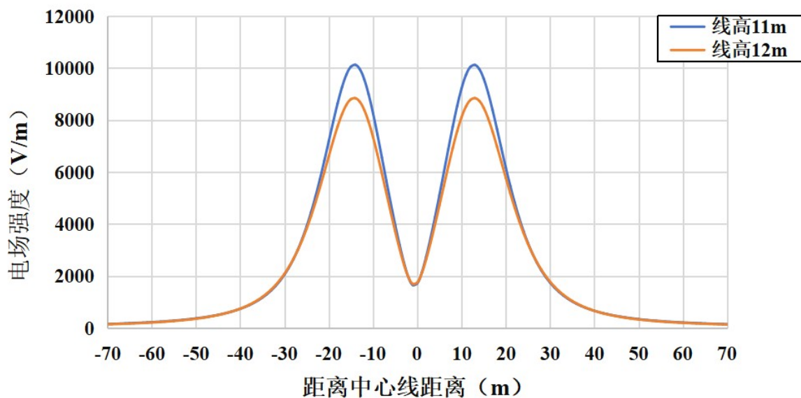
图 6-1 本线路通过耕地、园地等场所最不利塔型电场强度随距离变化趋势图
