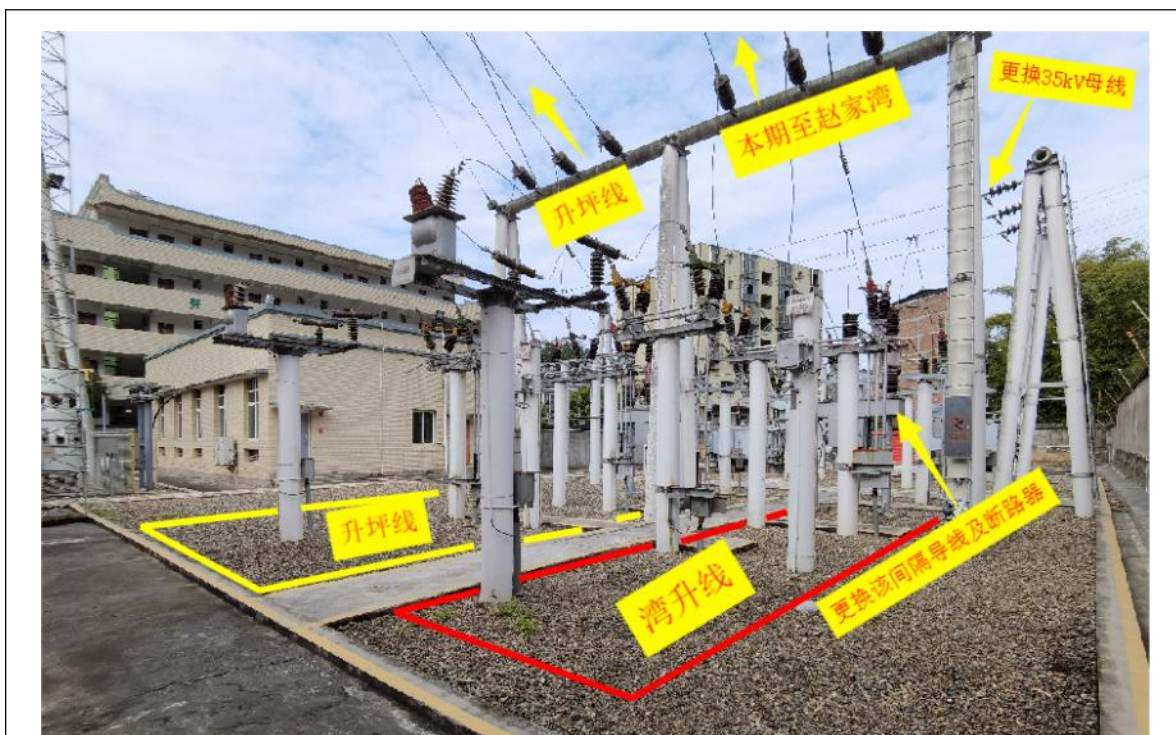
升钟站间隔改造更换导线示意图
