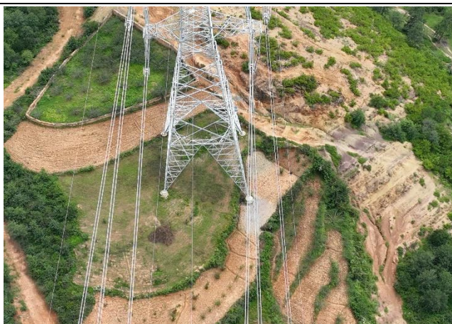
N7002塔基已实施植物措施
