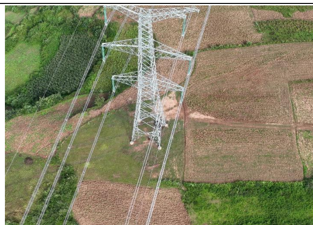
N2004塔基已实施植物措施
