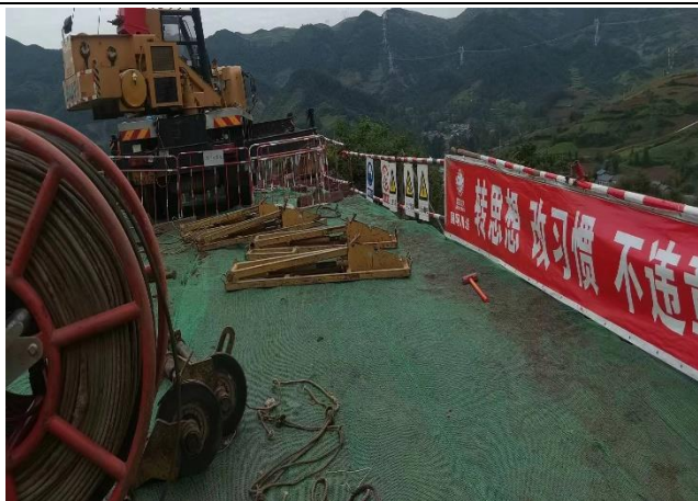
牵张场实施的临时防护措施
