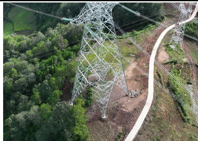
N2001塔基已架设完成并进行了场地平整
