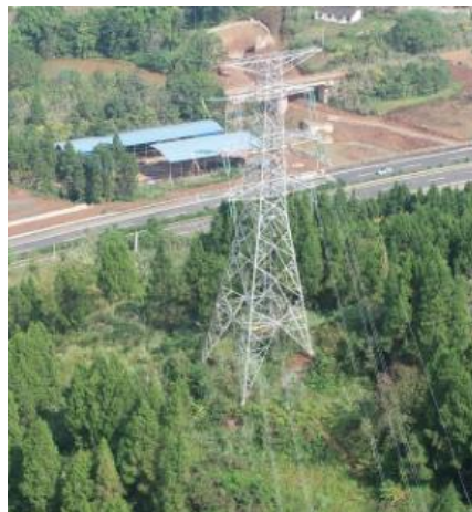
杨胡~灵泉 16#塔位
