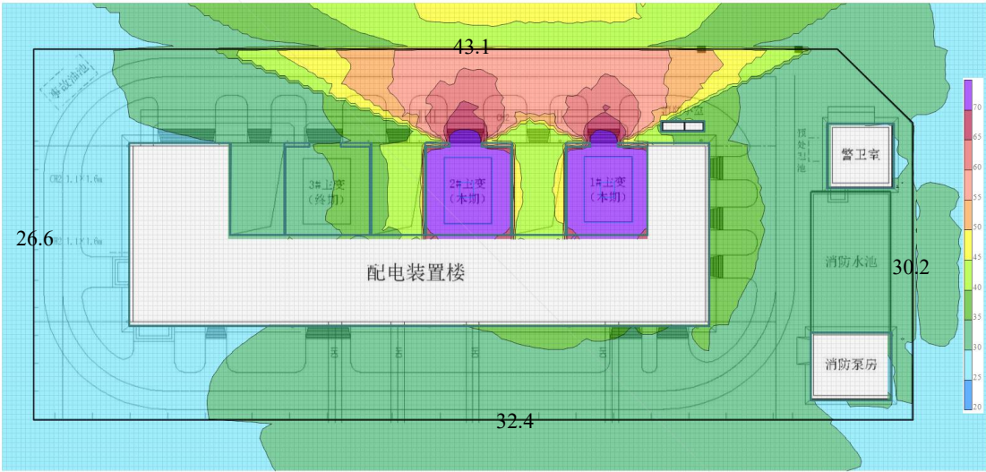
图 4-3 变电站本期规模运营期噪声贡献值等声级线图
