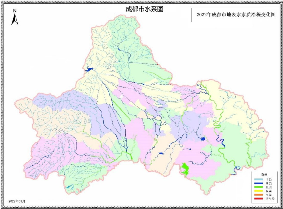
图 3-1 2022 年成都市地表水水质沿程变化图
