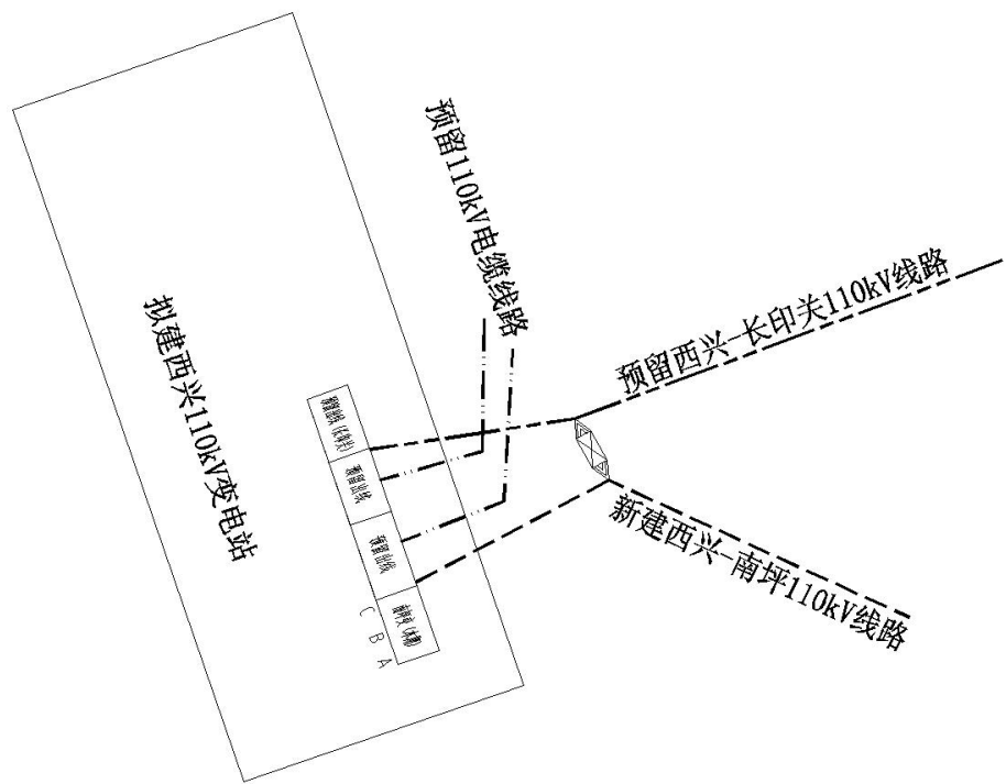
图 2.1-3 西兴 110kV 变电站间隔出线示意图
