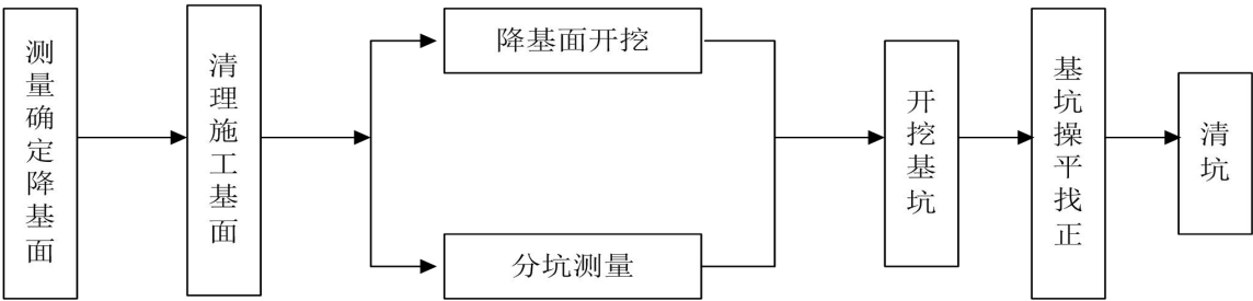
图 2.2-1 土石方施工流程
