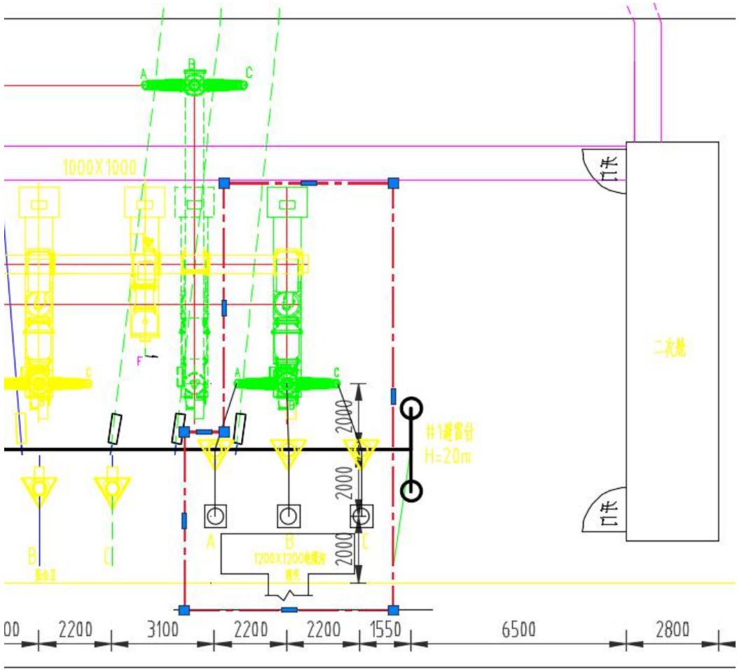
图 2.1-1 南坪 110kV 变电站西兴 110kV 间隔扩建工程平面图（红线框为扩建范围）
