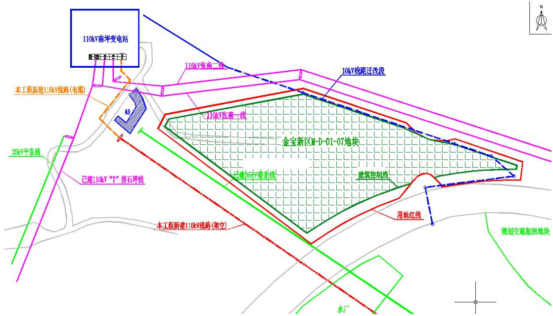
图 2.1-2 西兴 110kV 变电站端出线电缆和架空衔接段平面图
