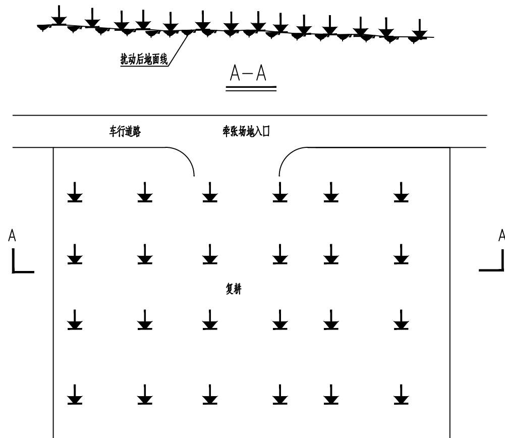
平面图(耕地)
