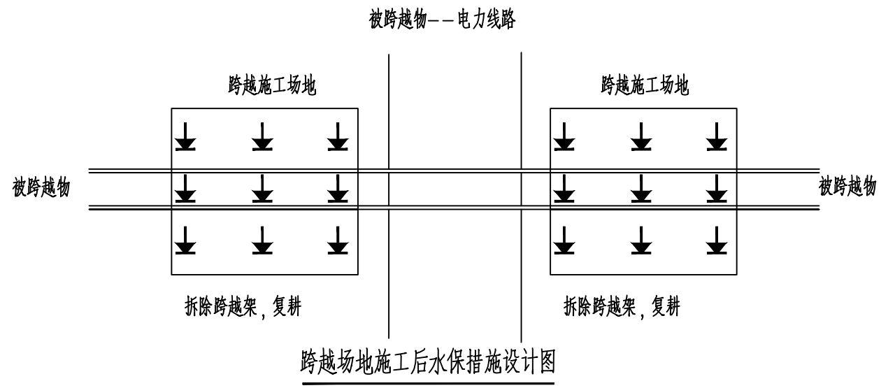
跨越场地施工后水保措施设计图
