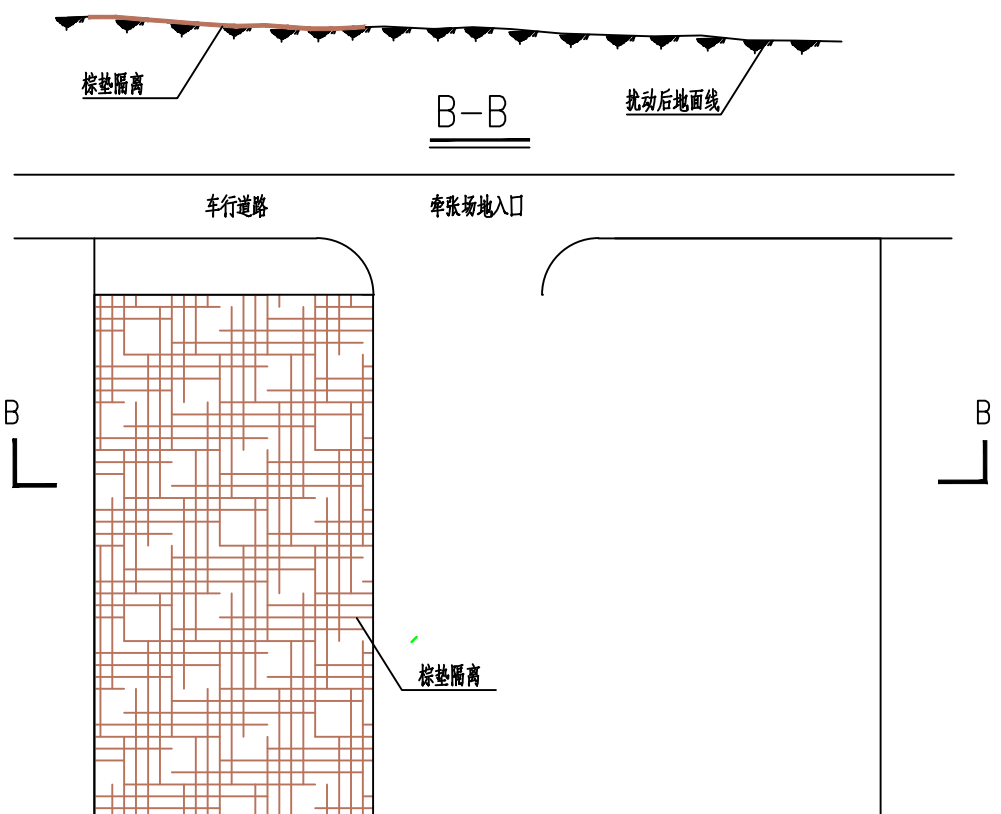
平面图(施工过程中)
