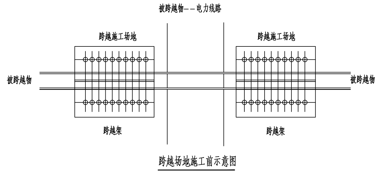
跨越场地施工前示意图
