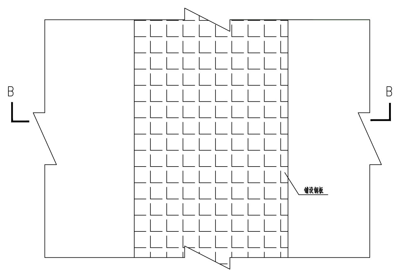
平面示意图(施工过程中)
