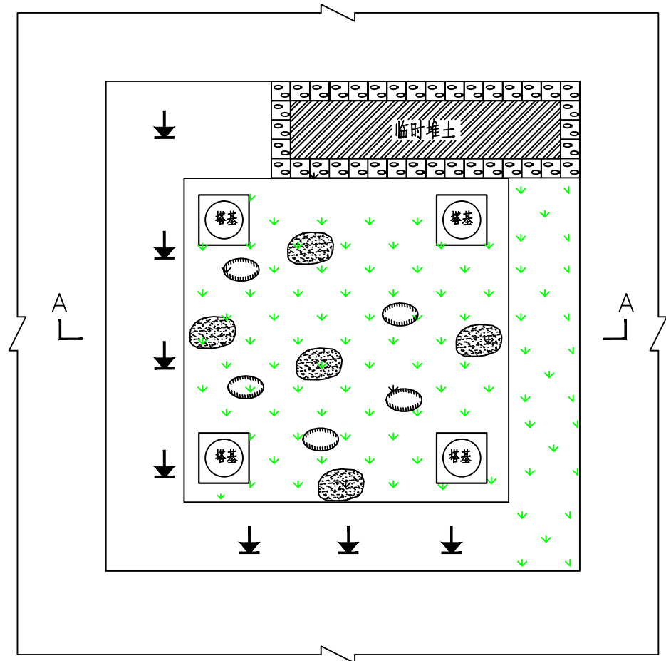
塔基水土保持措施布置图
