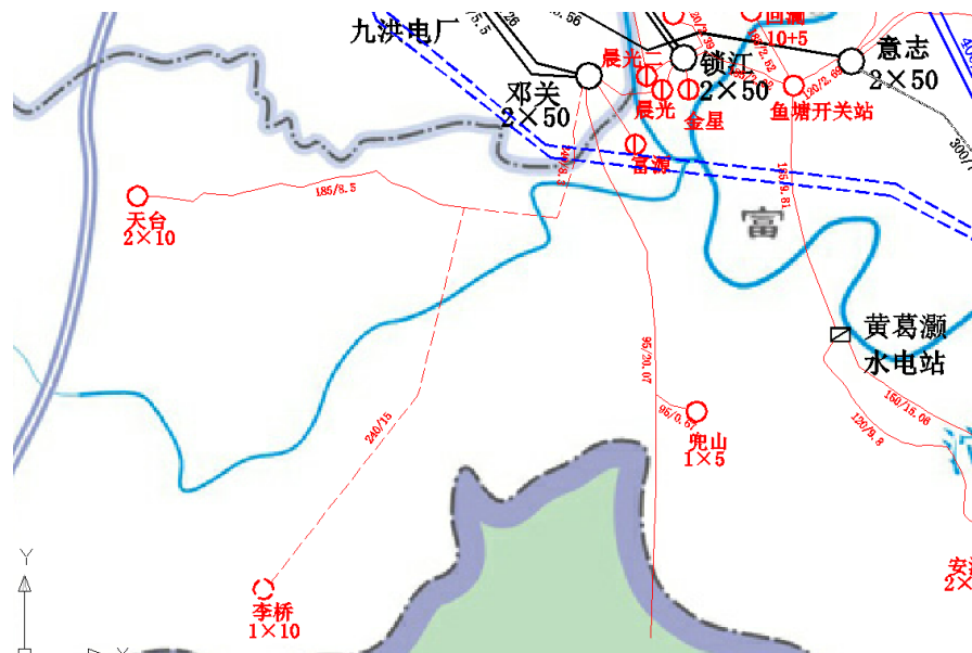
图 2.1-1 本项目变电站接入系统方案
