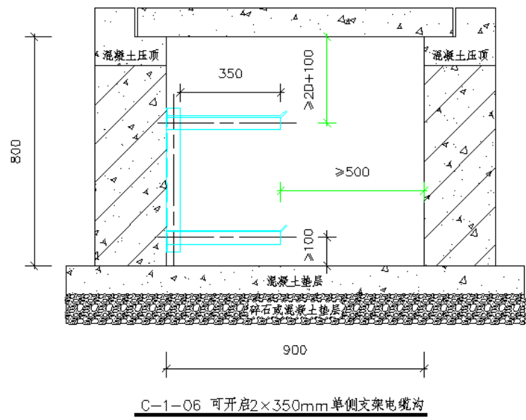
图 2.1-3 电缆沟截面图
