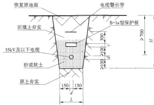
A-1-03 35kV及以下电缆单根敷设
